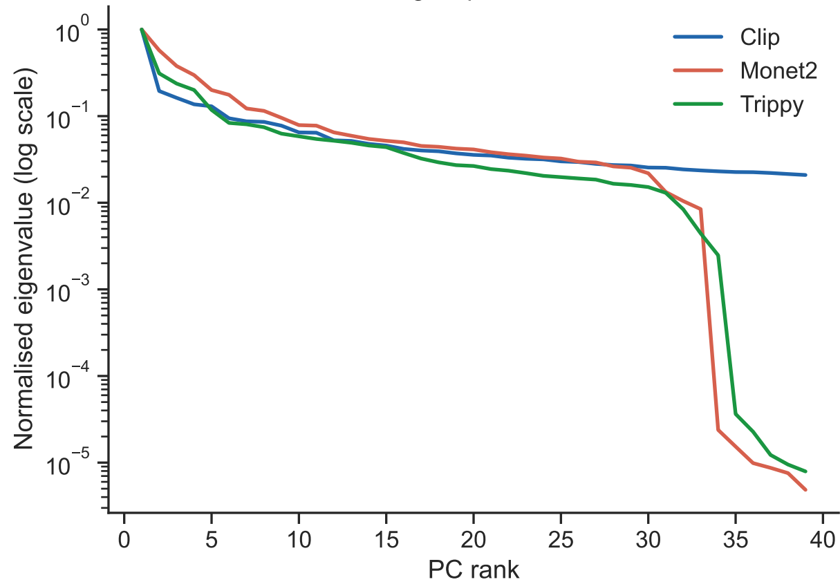
Eigenspectrum
