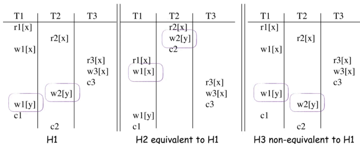
Figura 11.7: Esempio di uno schedule H_2 equivalente ad H_1 e di uno schedule H_3 non equivalente ad H_1
