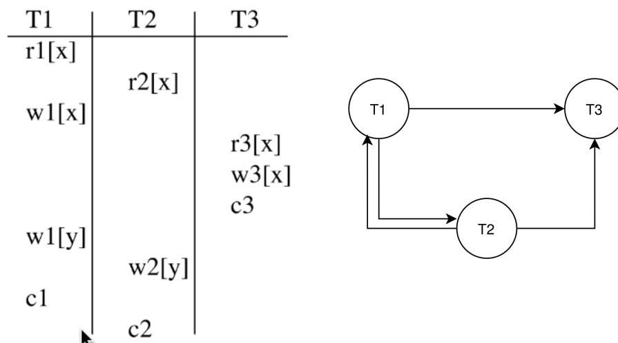
Figura 11.8: Esempio di grafo di precedenza dato uno schedule H
