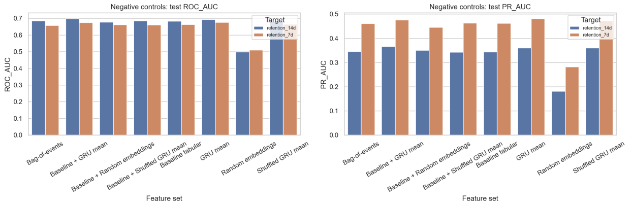
Рисунок 2 – Сравнение RNN-эмбедингов с отрицательными контролями на тестовой части.
