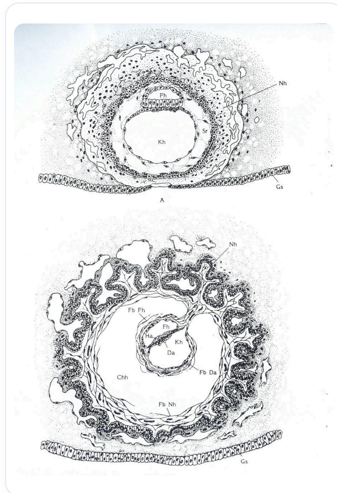
ABB. — Kalziumsalze
