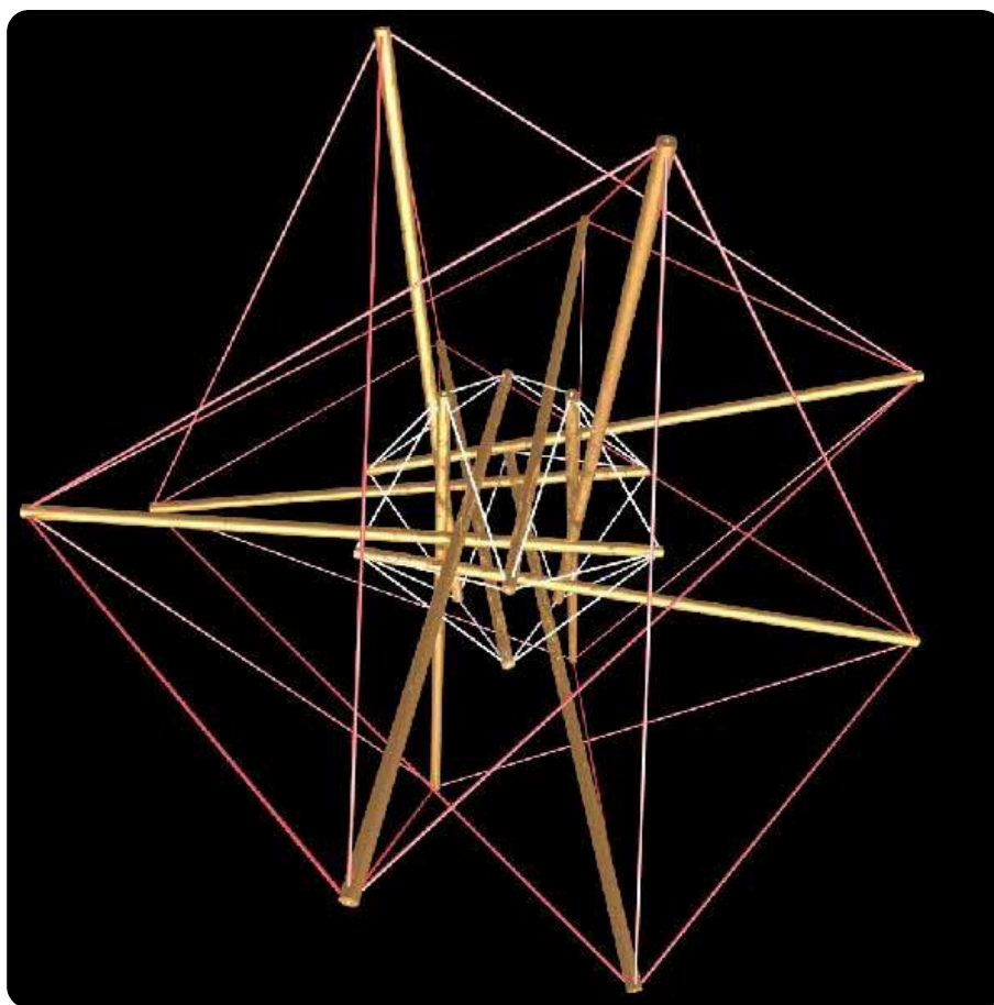
FIG. — Struttura a tensgheità
