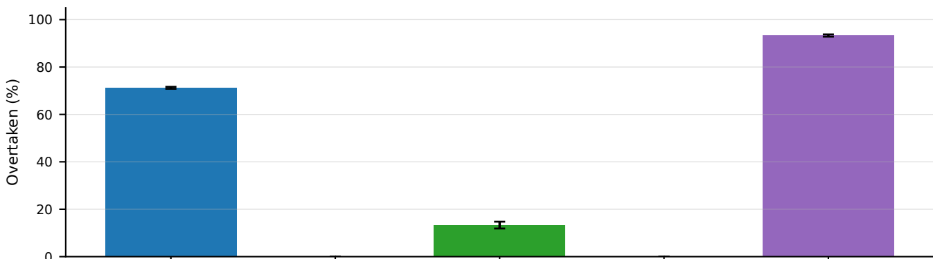
Unseen
