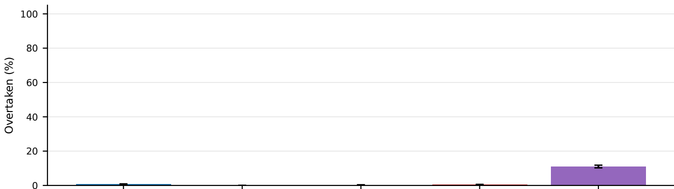
Unseen
