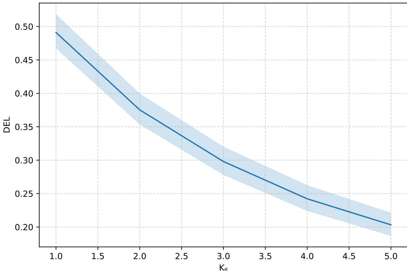
DEL with 95% CI — COSINE
