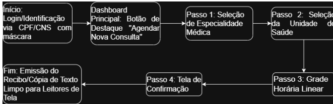
Fig. 1: Fluxograma detalhado mostrando as etapas sequenciais desde o Login via CPF/CNS, passando pelas telas de seleção de especialidade, UBS, grade horária, até a tela de confirmação e impressão do recibo acessível.
