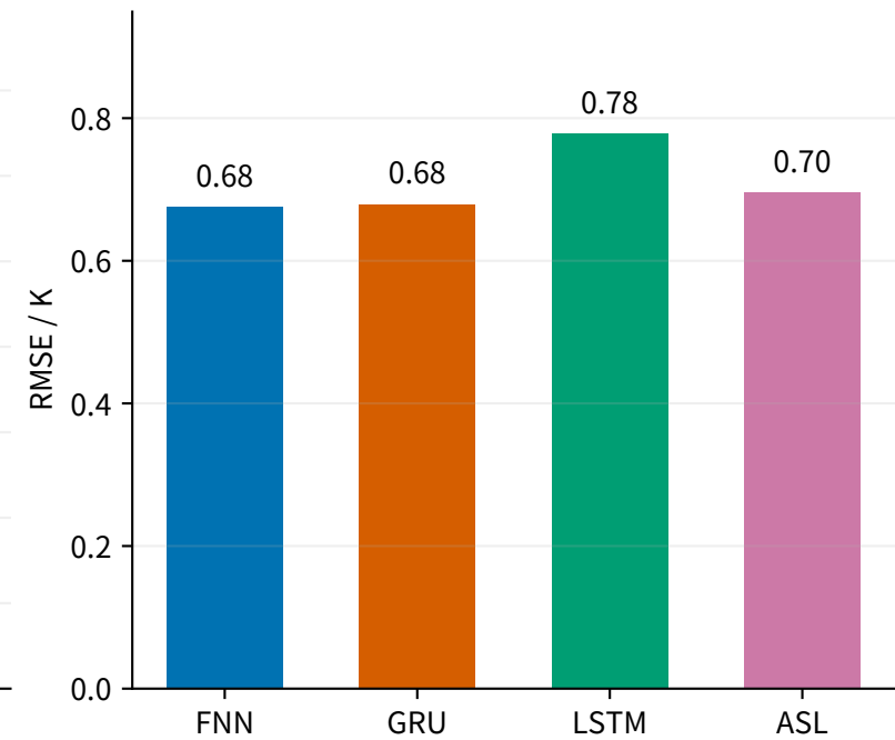
冷端实验测试误差
