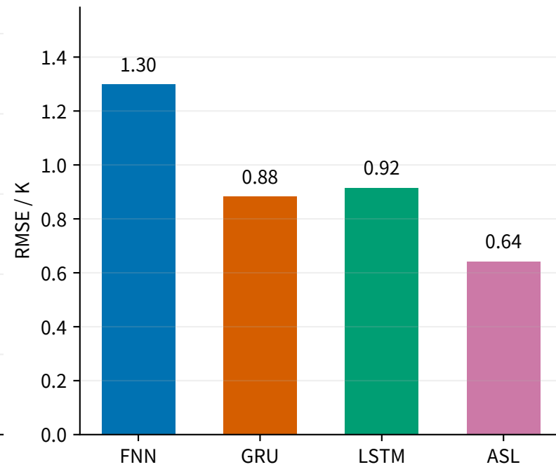
热端实验测试误差
