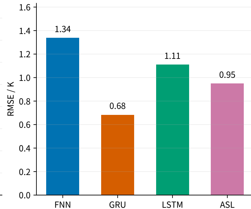
热端实验测试误差
