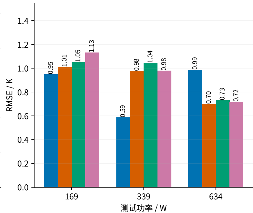
冷端：各测试功率
