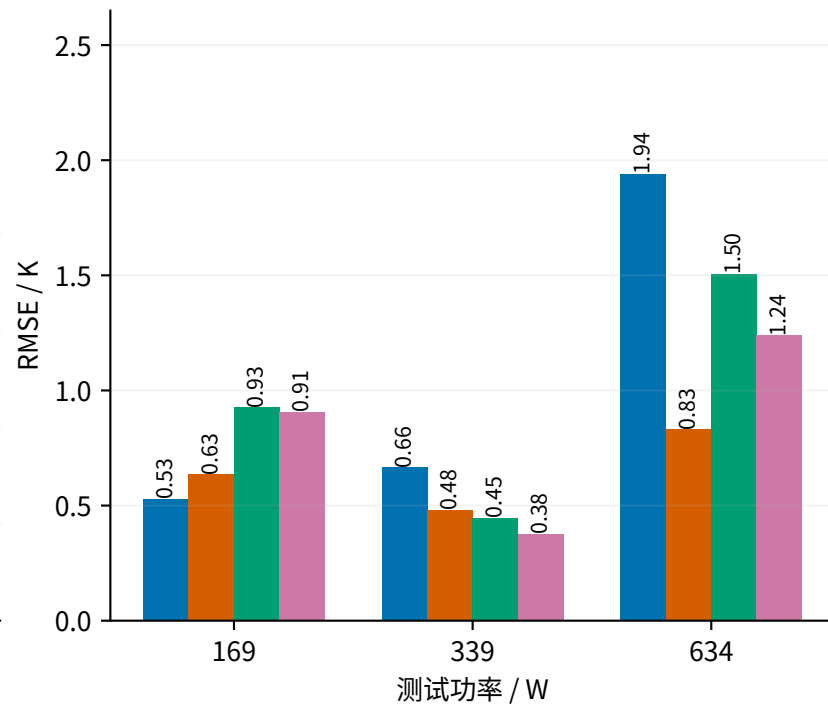
热端：各测试功率
