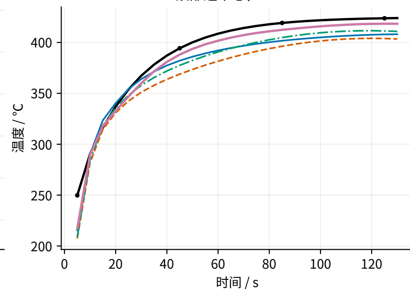
热端, 634 W
