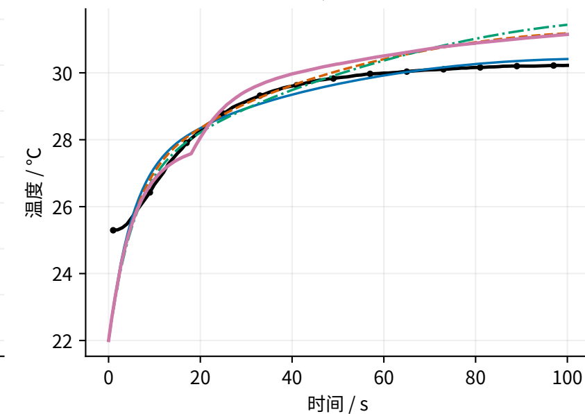
冷端, 339 W
