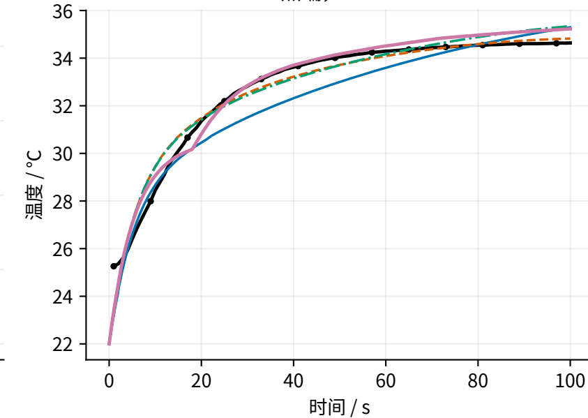
冷端, 339 W
