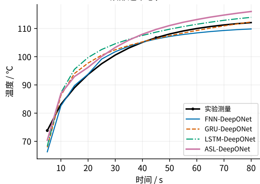
热端, 169 W
