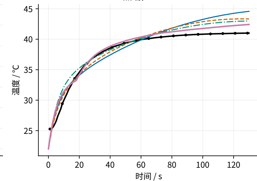
冷端, 634 W
