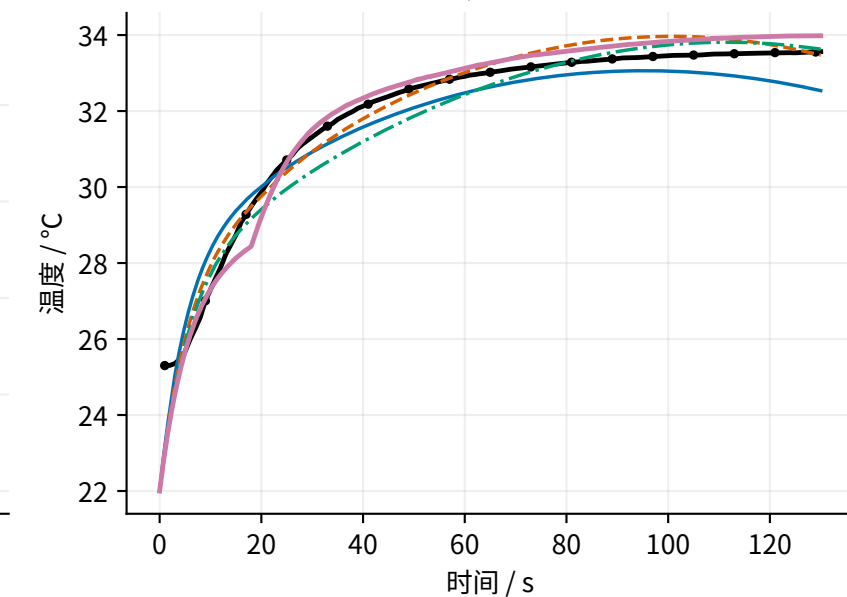
冷端, 634 W
