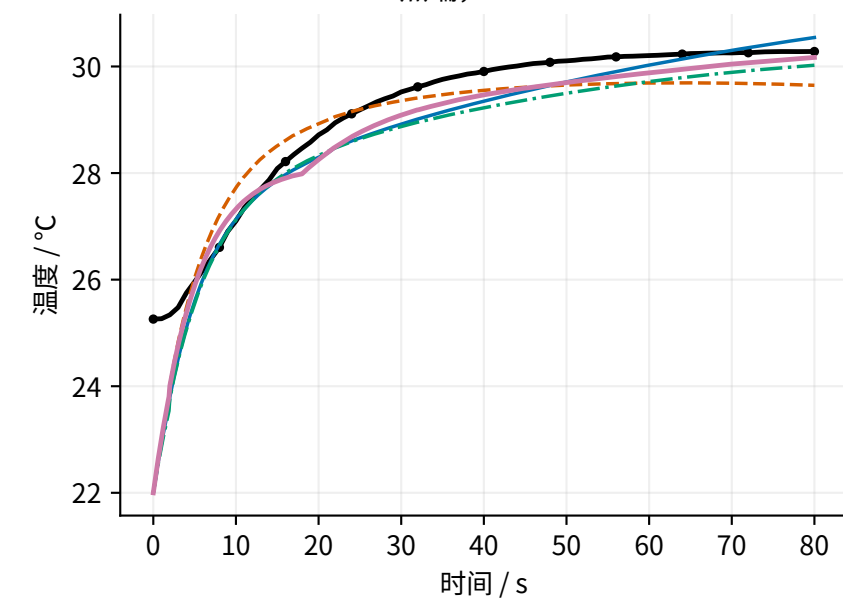
冷端, 169 W
