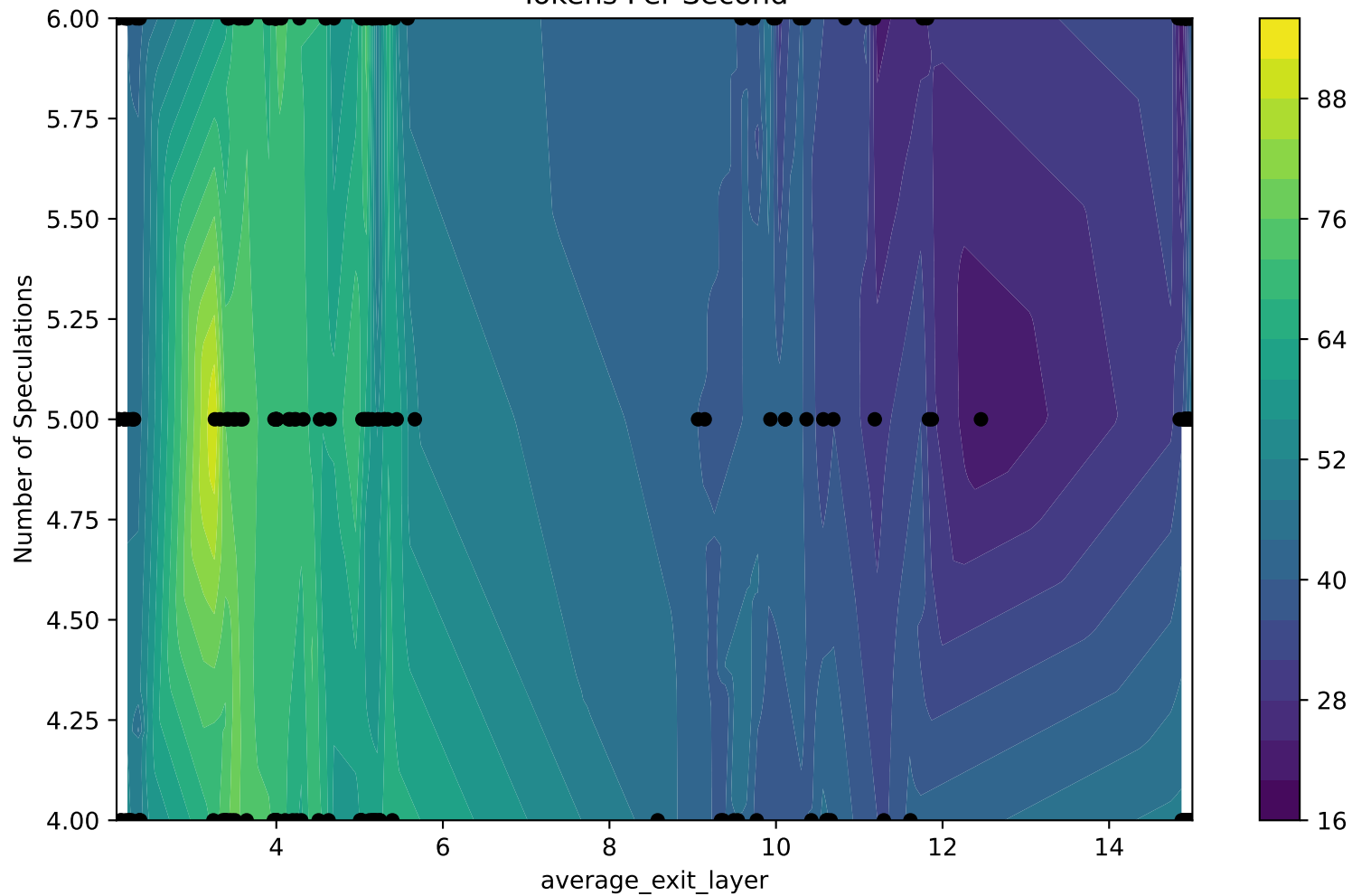
Tokens Per Second
