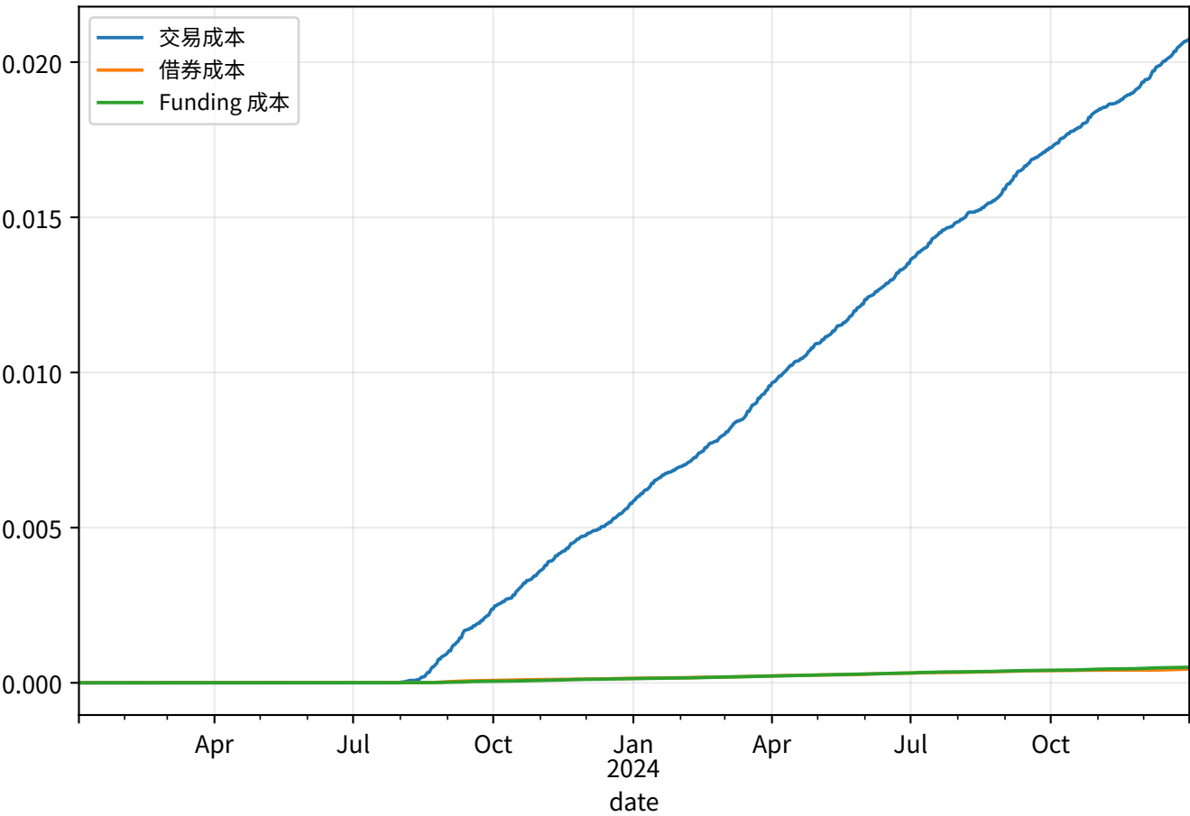
累计成本
