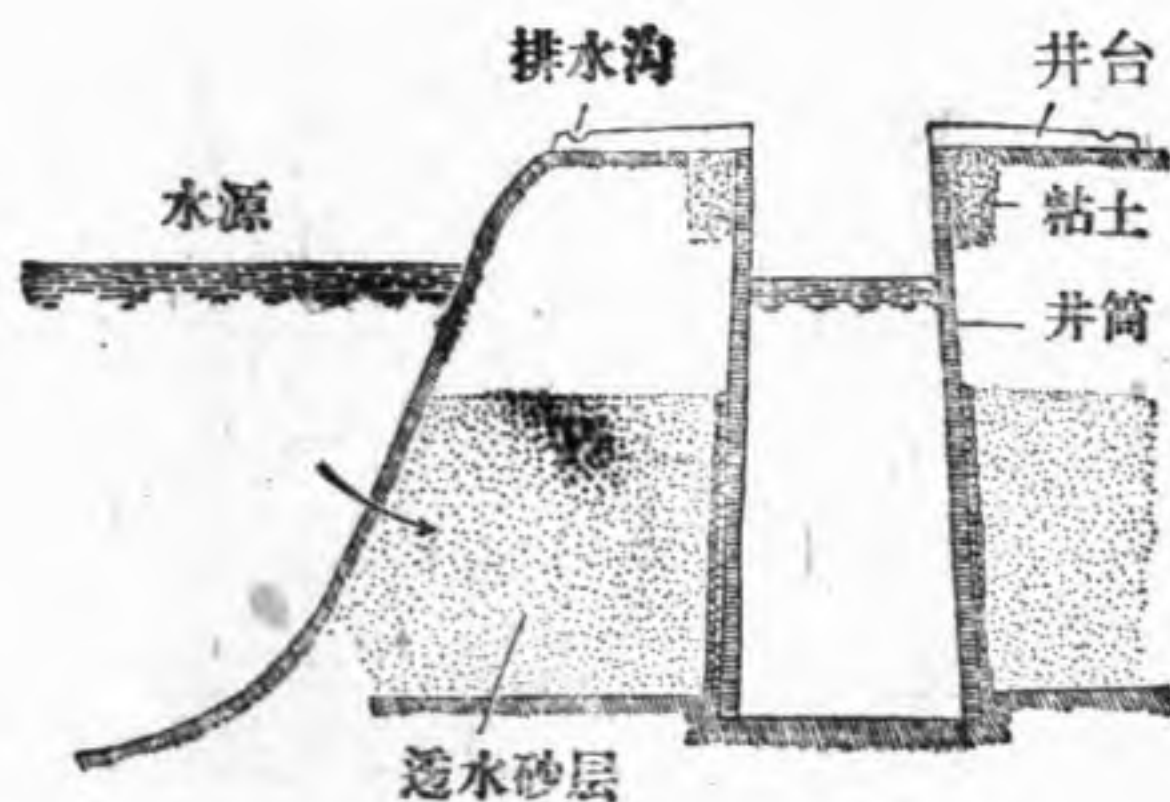
图 2 ~ 3 滤水井示意图
