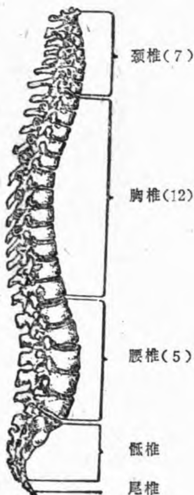
图3～5 脊柱
