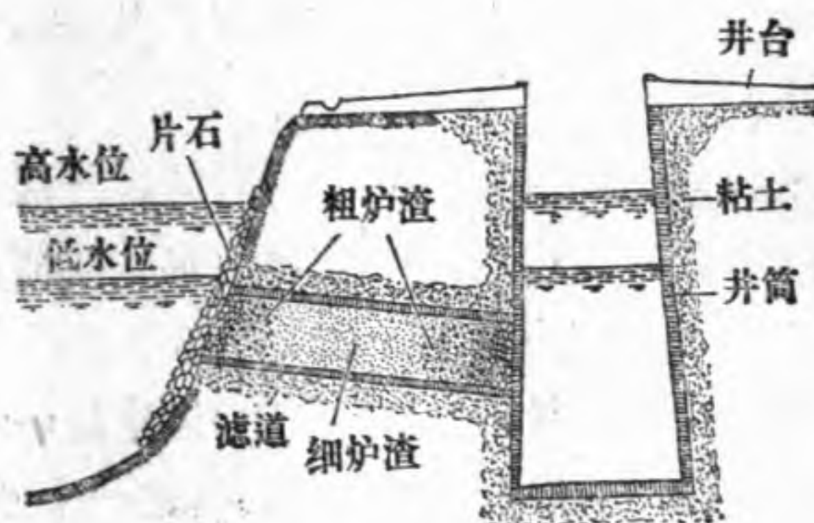
图 2 ~ 4 沙滤井示意图
