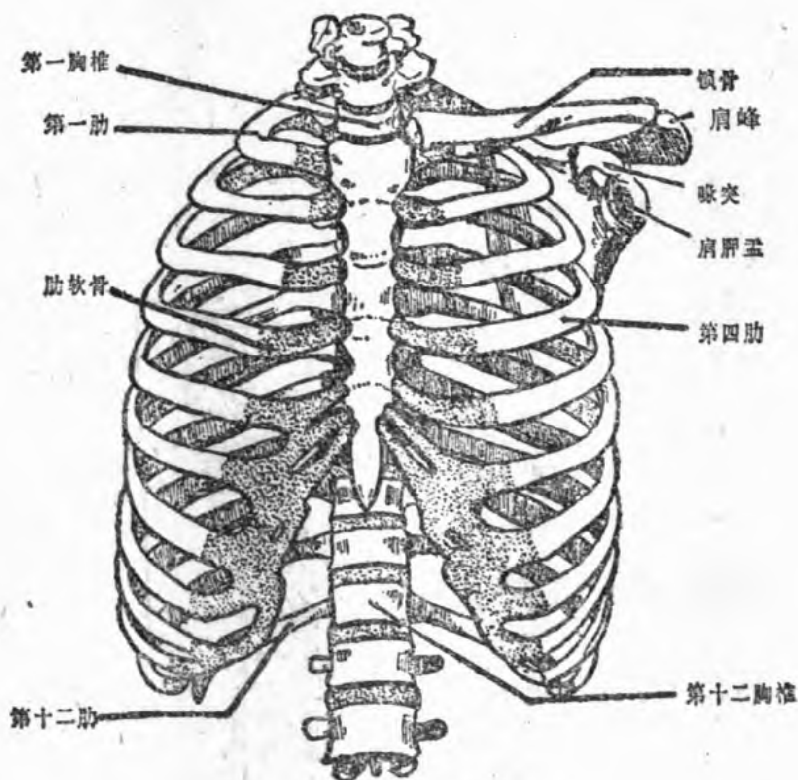
图3~6 胸廓正面图
