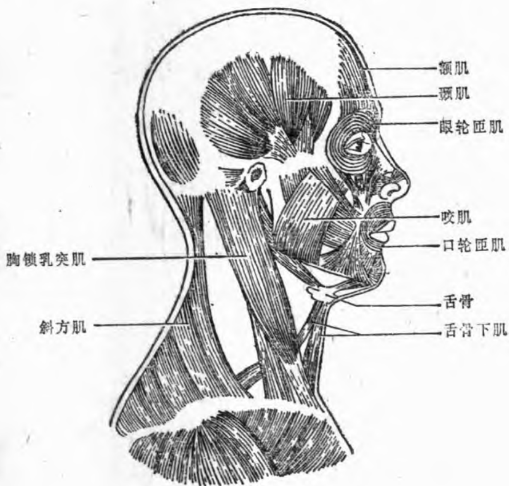
图3~9 头颈部肌肉
