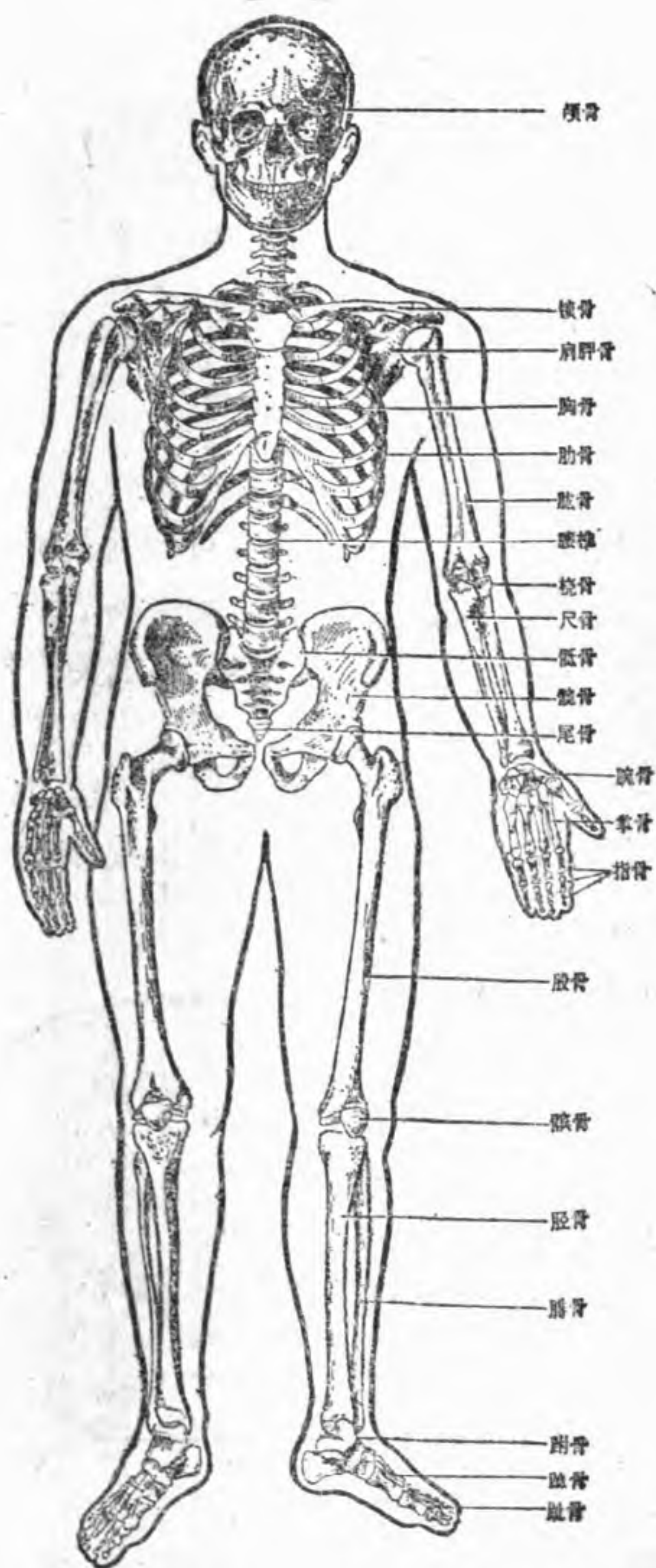
图 3~1 人体骨骼图
