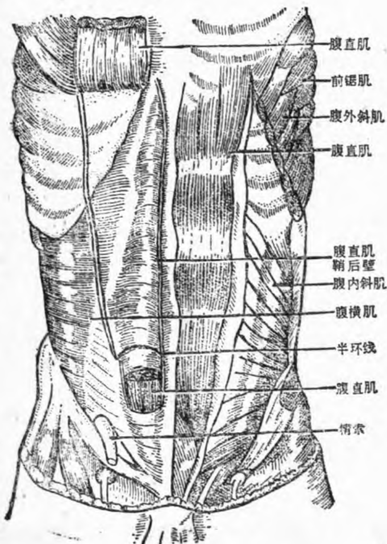
图 3 ~ 13 腹壁肌肉
