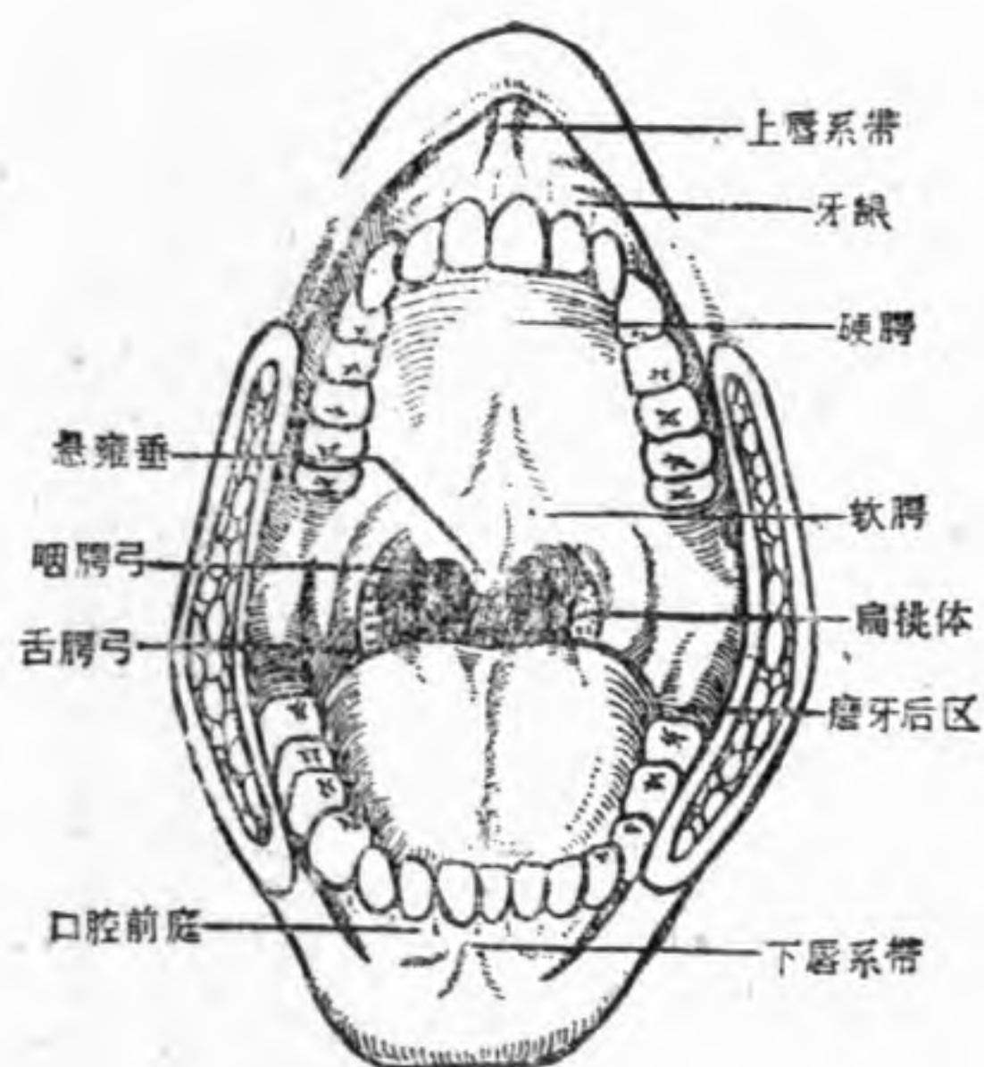
图 3~17 口 腔
