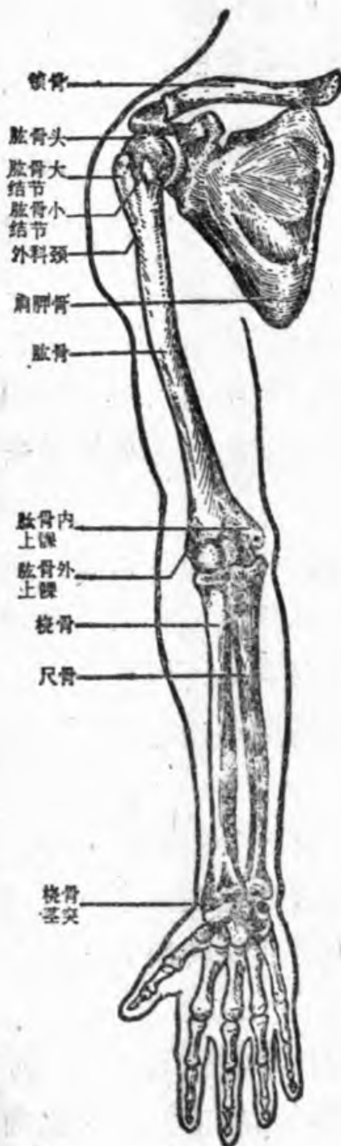
图 3~7 上肢骨
