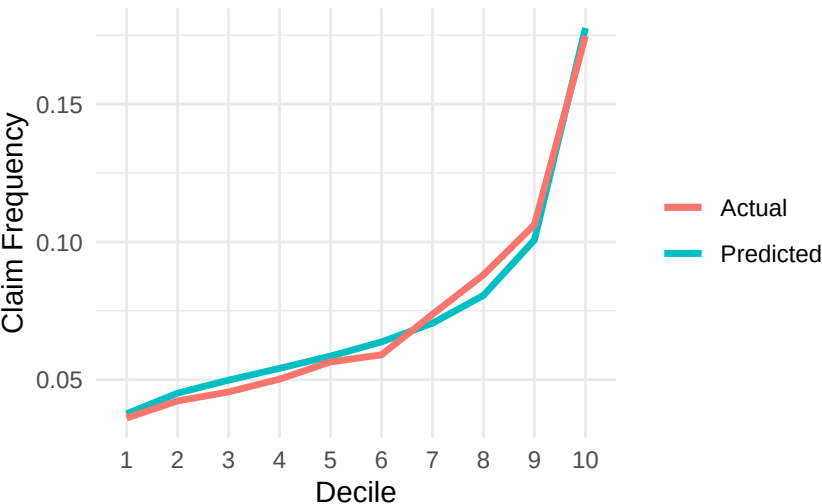
Decile Plot: Actual vs Predicted (Test Set)
