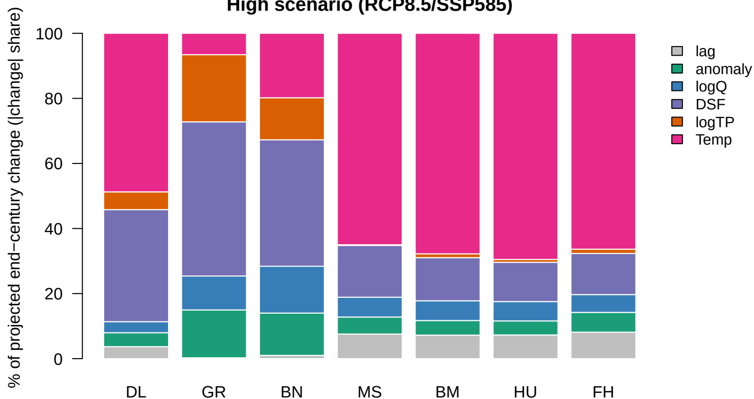
High scenario (RCP8.5/SSP585)
