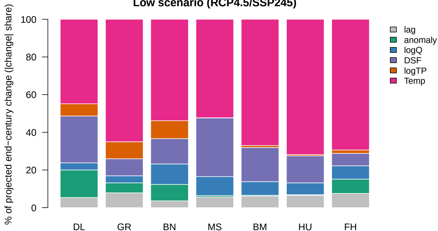
Low scenario (RCP4.5/SSP245)
