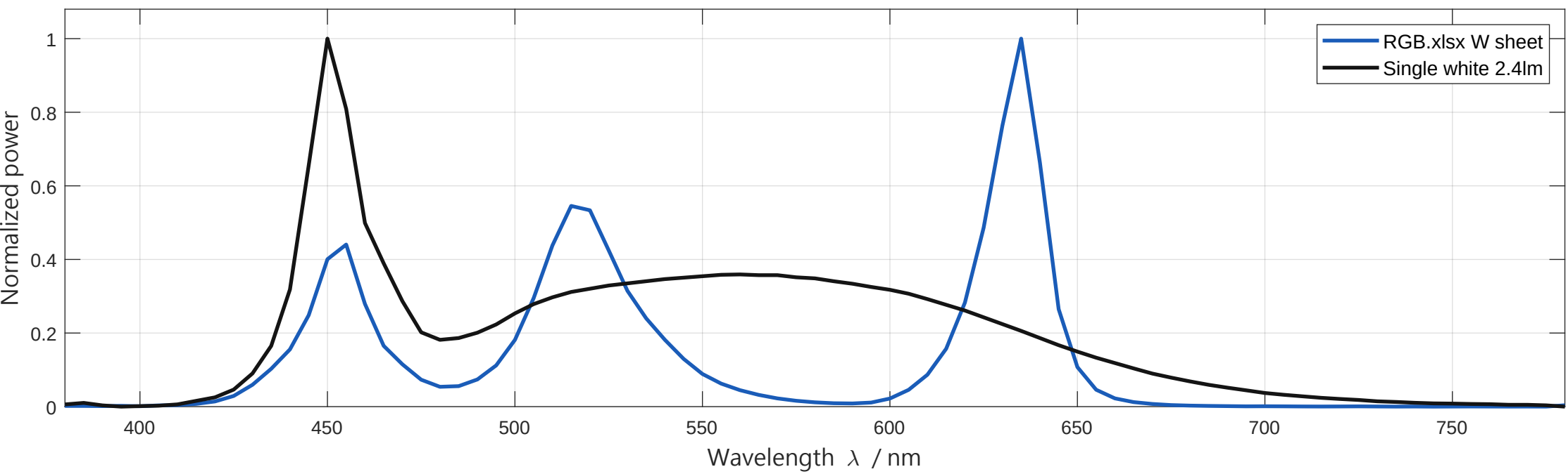
RGB.xlsx W sheet 与单白灯输入光谱
