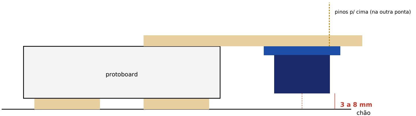
JEITO B · pinos saem para CIMA ou para o lado: palito em cima da protoboard, módulo embaixo da ponta
