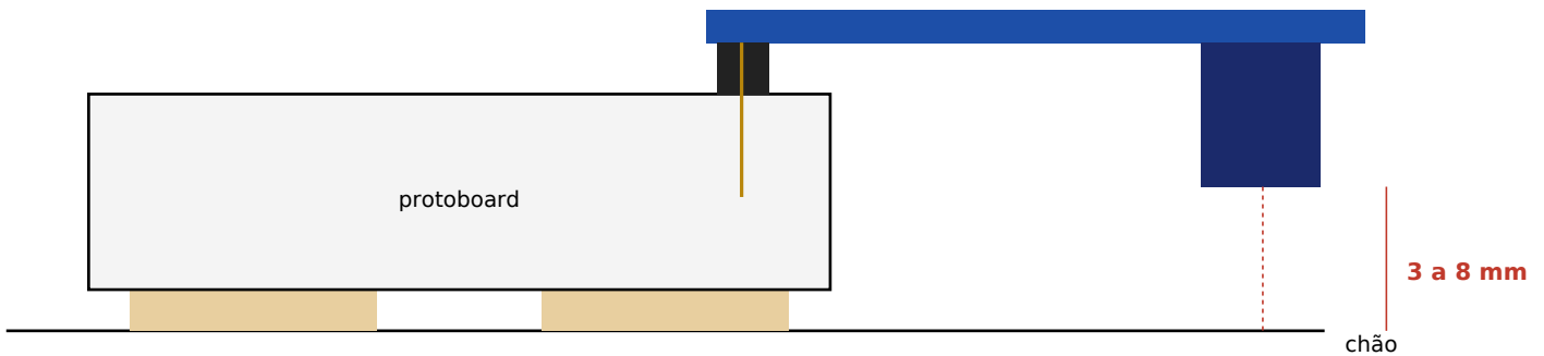
JEITO A · pinos saem para BAIXO (mesmo lado do sensor): espete direto na protoboard
