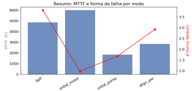
Figura 4. Resumo dos quatro modos com eixo Y duplo: MTTF em horas (barras azuis, referenciadas no eixo esquerdo) e parâmetro de forma \beta da Weibull (linha vermelha com marcadores circulares, referenciada no eixo direito). A linha cinza pontilhada em \beta = 1 demarca a transição entre falha por taxa constante e desgaste.
