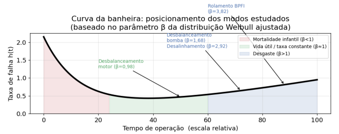
Figura 6. Curva da banheira com o posicionamento dos quatro modos segundo o parâmetro de forma \beta da Weibull ajustada. A zona de mortalidade infantil ( \beta < 1 ) não possui anotações pois nenhum modo mecânico progressivo se comporta como falha prematura de partida. O desbalanceamento no motor ( \beta \approx 1 ) situa-se na vida útil (taxa de falha constante), enquanto os demais modos representam falhas de desgaste ( \beta > 1 ).
