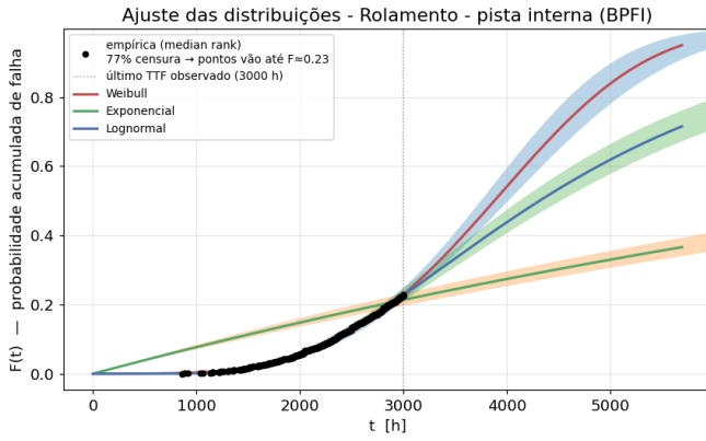
Figura 2. Ajuste das distribuições sobre a CDF do rolamento BPFI. Os pontos pretos (empírica) terminam em F \approx 0,23 porque 77% das unidades simuladas foram censuradas à direita (não falharam até o horizonte de observação); os modelos extrapolam além desse ponto usando a informação das censuras. A Exponencial (verde) se afasta cedo pois assume falha imediata desde t=0 , enquanto Weibull e Log-normal capturam o onset tardio das falhas de desgaste. A linha pontilhada marca o último TTF observado (3000 h).
