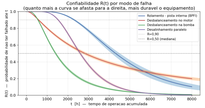
Figura 5. Confiabilidade R(t) dos quatro modos de falha: a curva mais à direita representa o modo mais durável. O desbalanceamento na bomba (verde) é o modo mais crítico — metade das unidades falham antes de 1100 h. O rolamento BPFI (azul) é o mais robusto, com MTTF de 4857 h. As bandas coloridas são os IC 95% por bootstrap .
