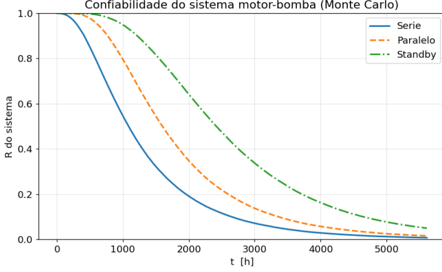
Figura 7. Confiabilidade R(t) do sistema motor-bomba por Monte Carlo nas três configurações. A ordenação standby > paralelo > série é a esperada.
