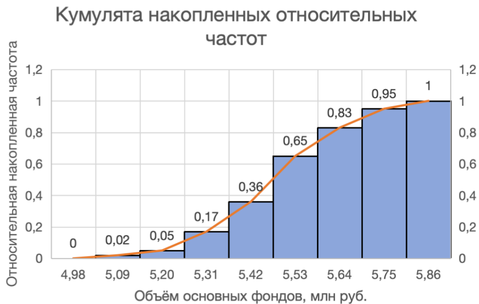
Рис. 6 – Кумулята накопленных относительных частот
