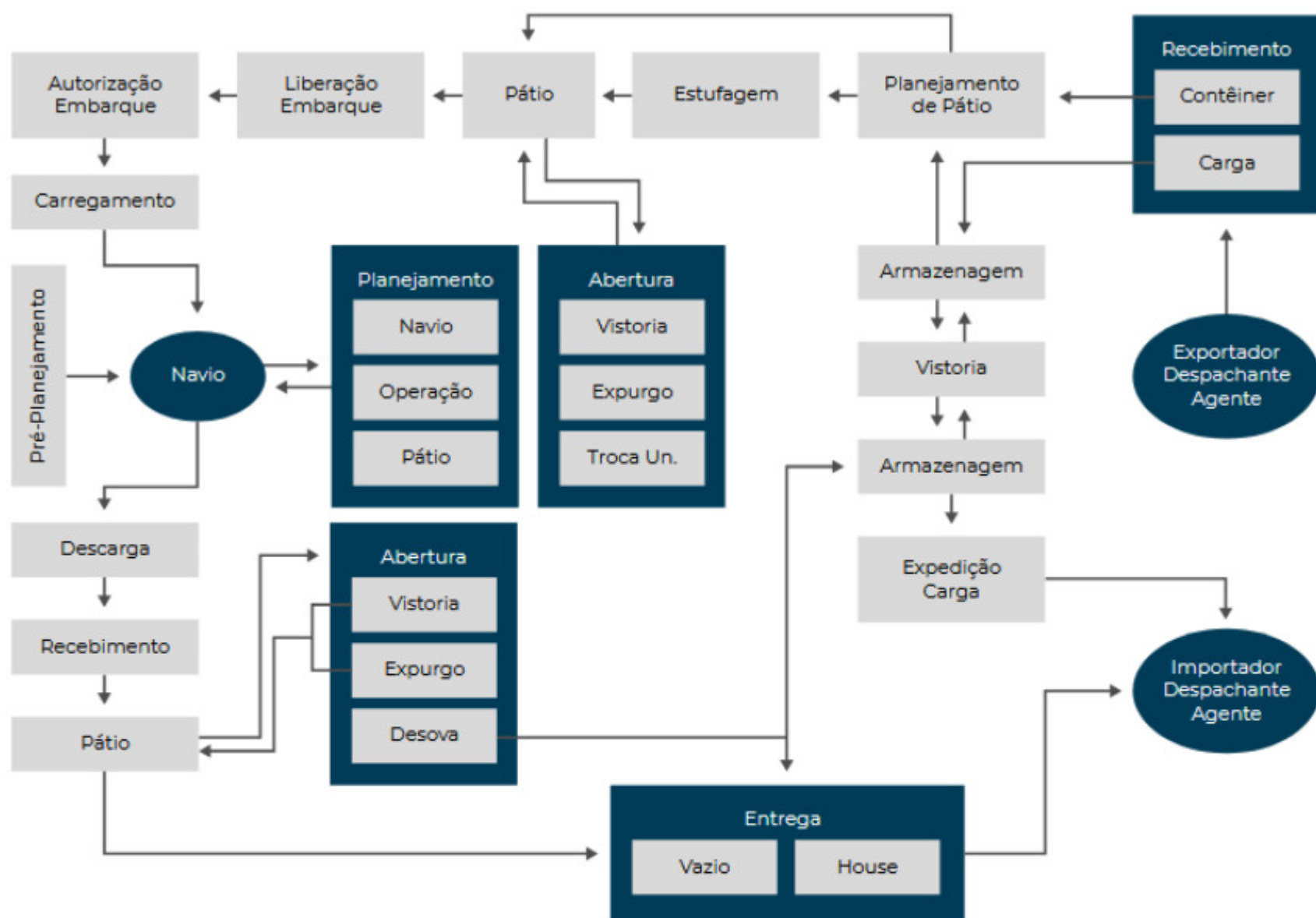
Figura 1 - Fluxograma completo das operações portuárias de embarque e desembarque de mercadorias
