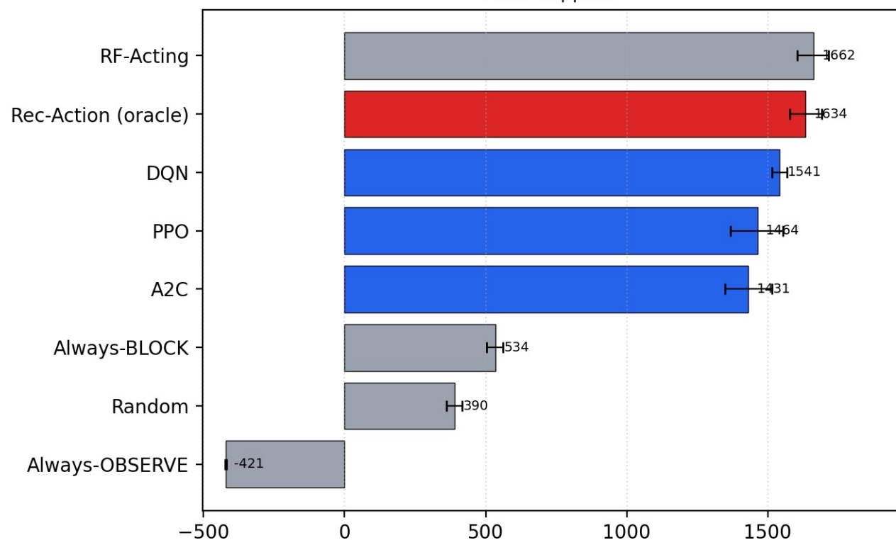
XSS
