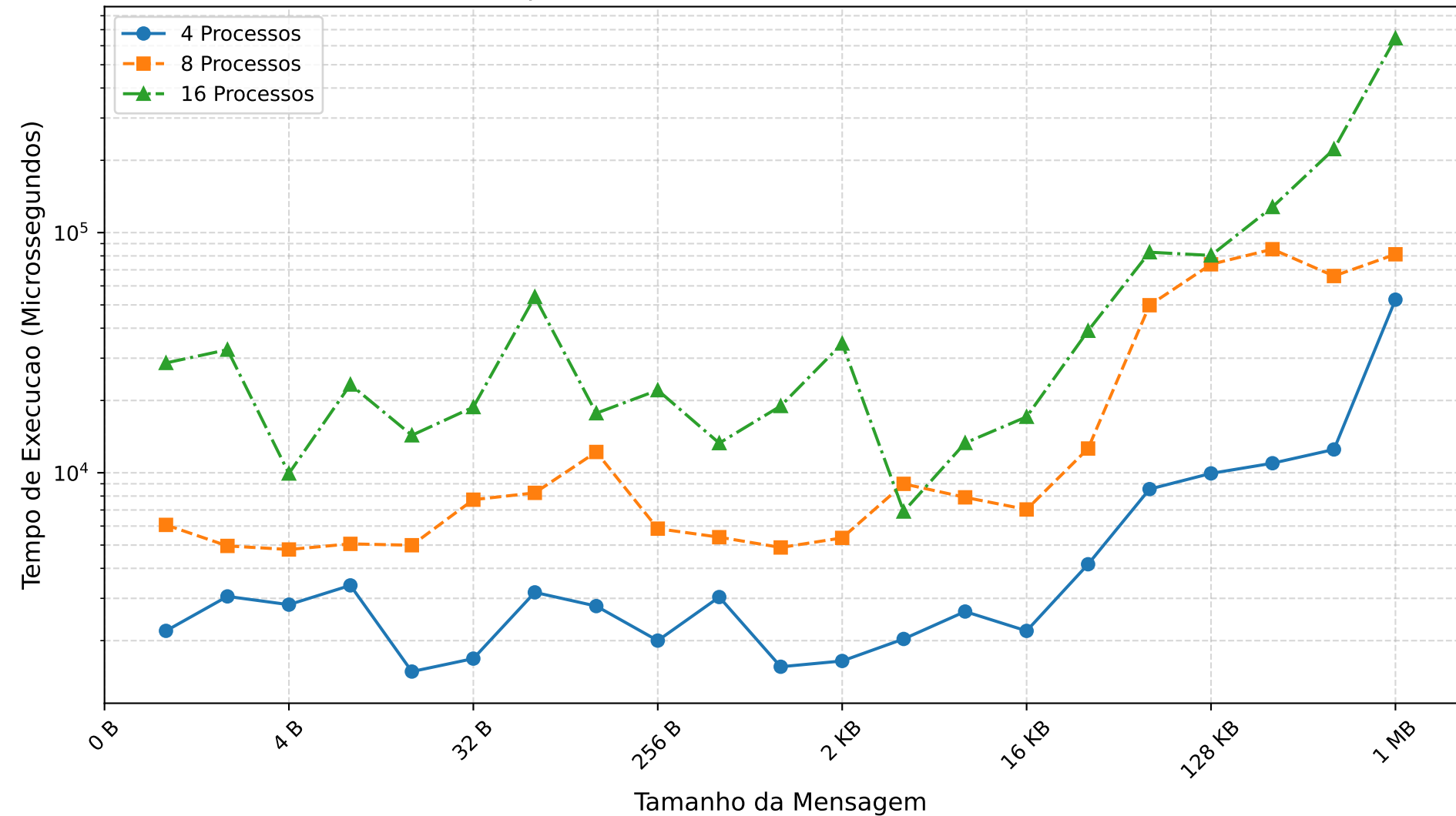
Desempenho de Broadcast no VirtualBox (4 VMs)
