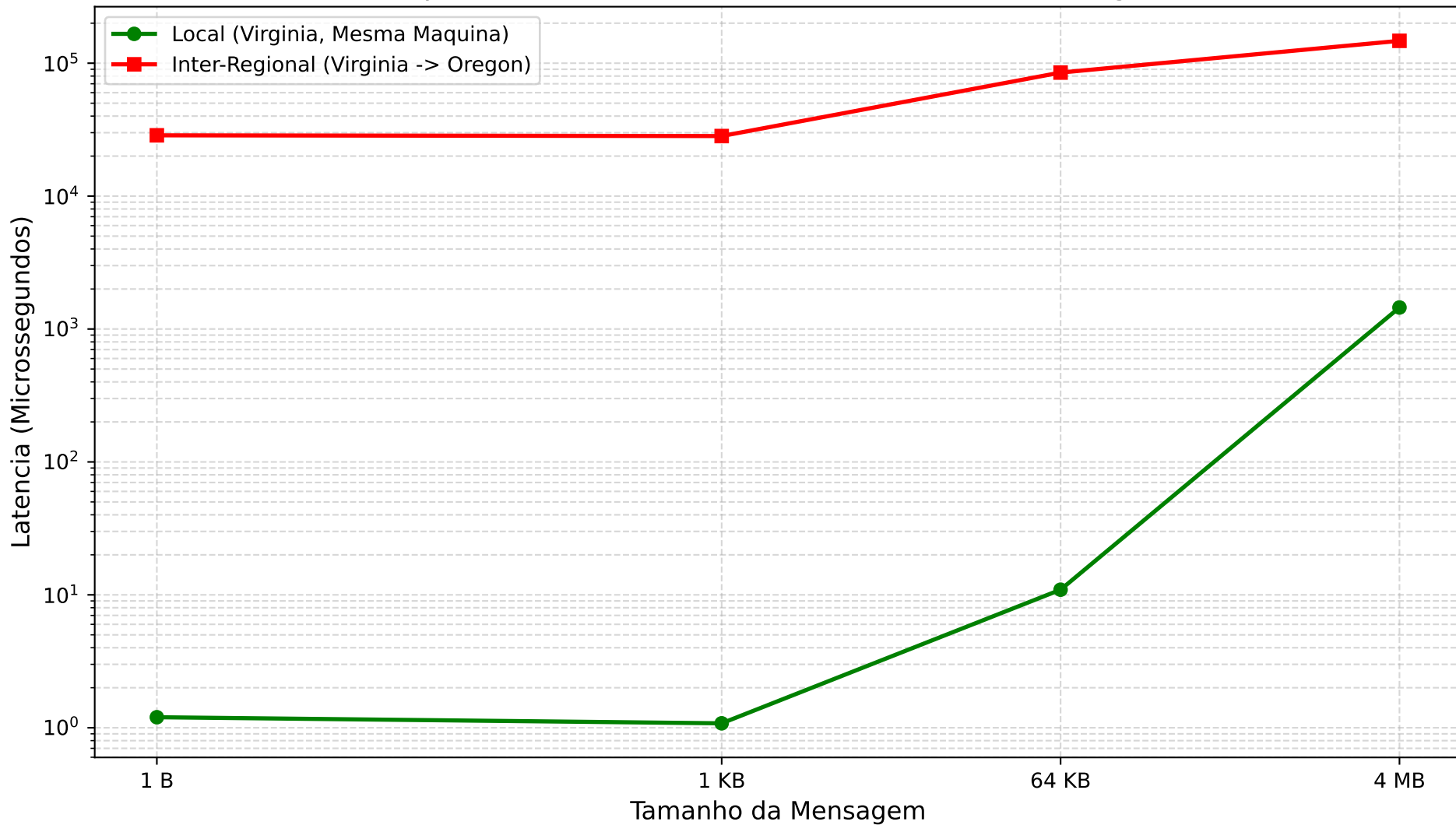
Comparativo de Latencia na AWS: Local vs. Inter-Regional
