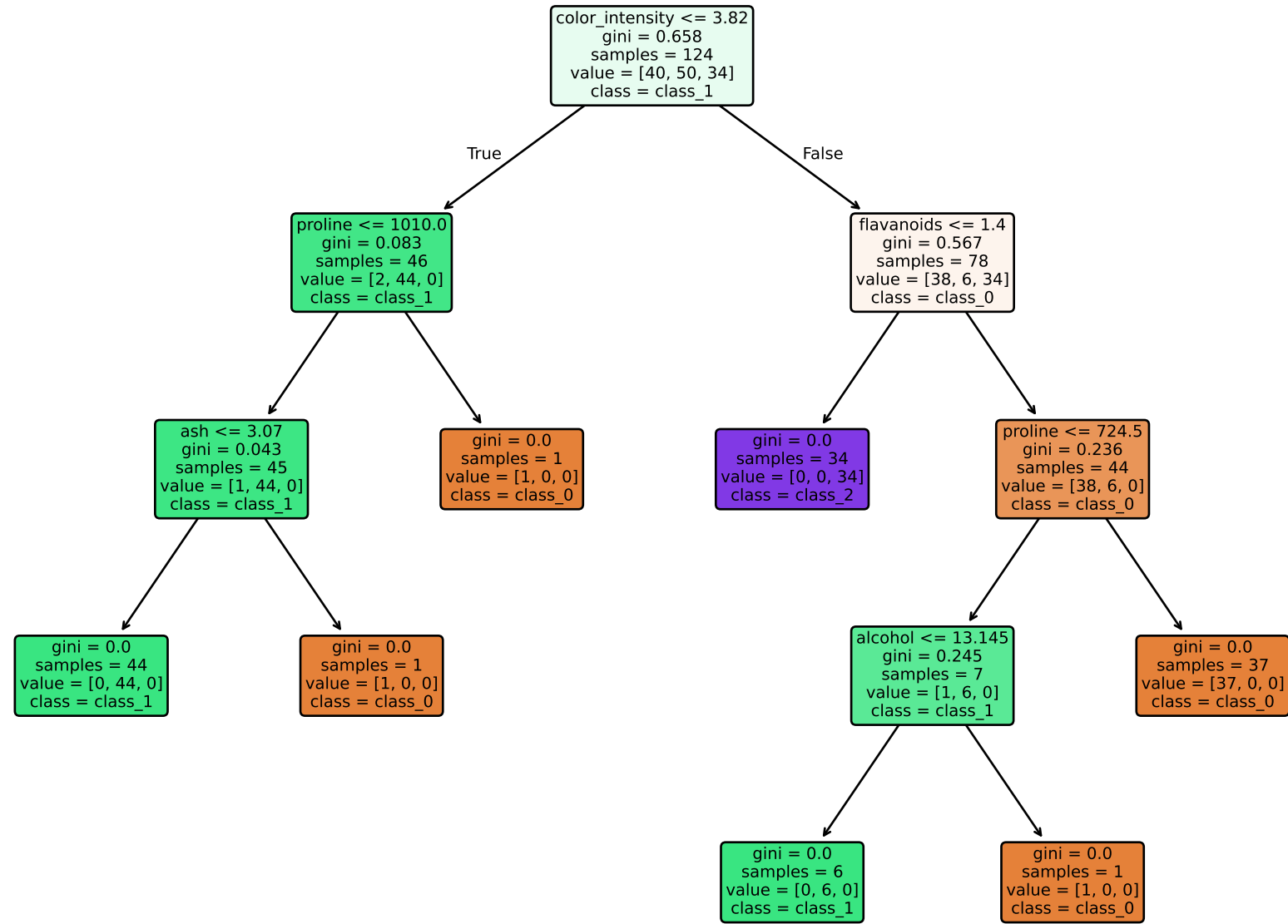
Árvore de Decisão completa
