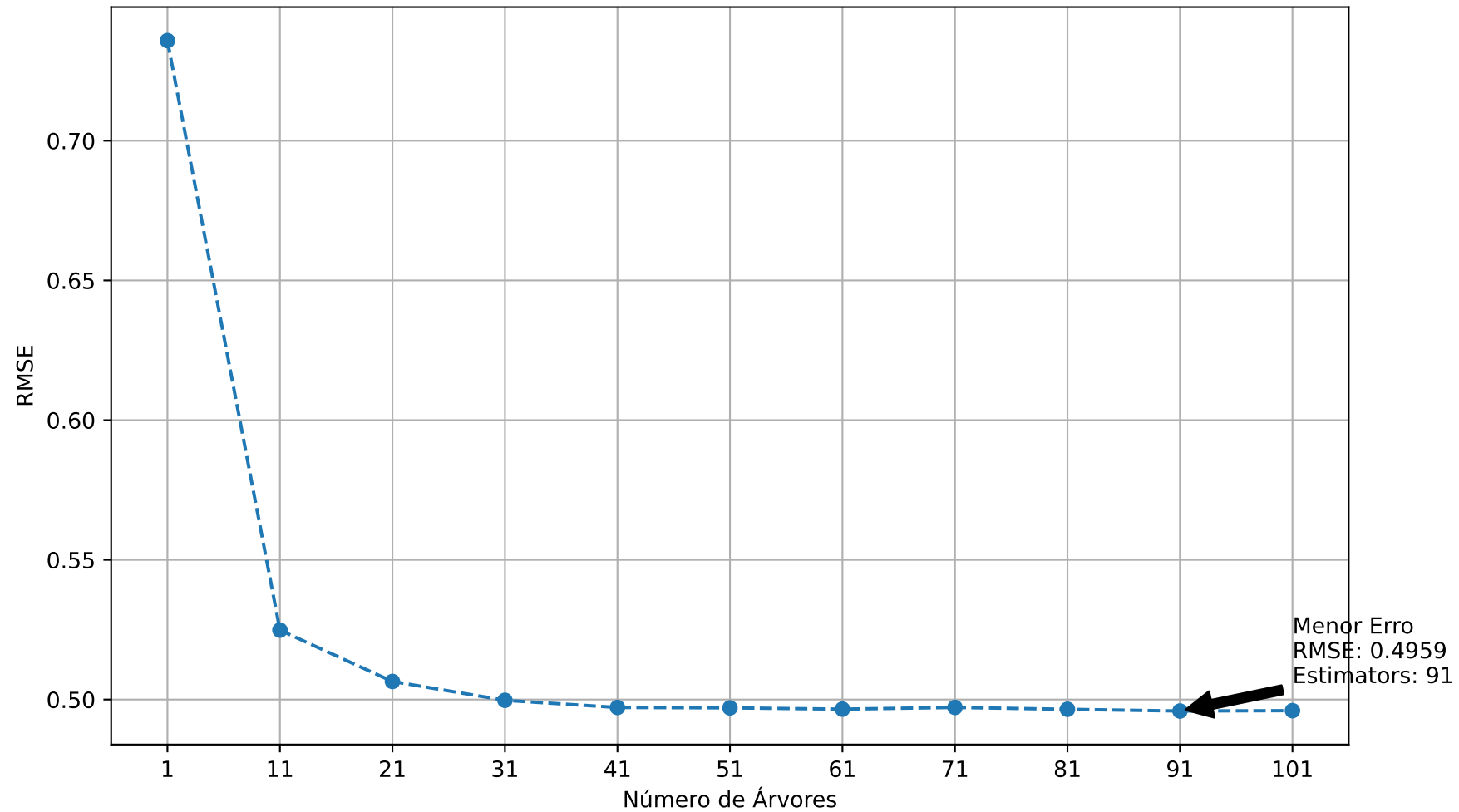
RMSE do Modelo vs. Número de Árvores na Floresta
