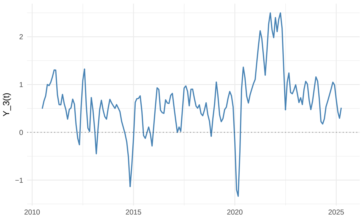
yout[, h=3]: cumulativo 3-passos
