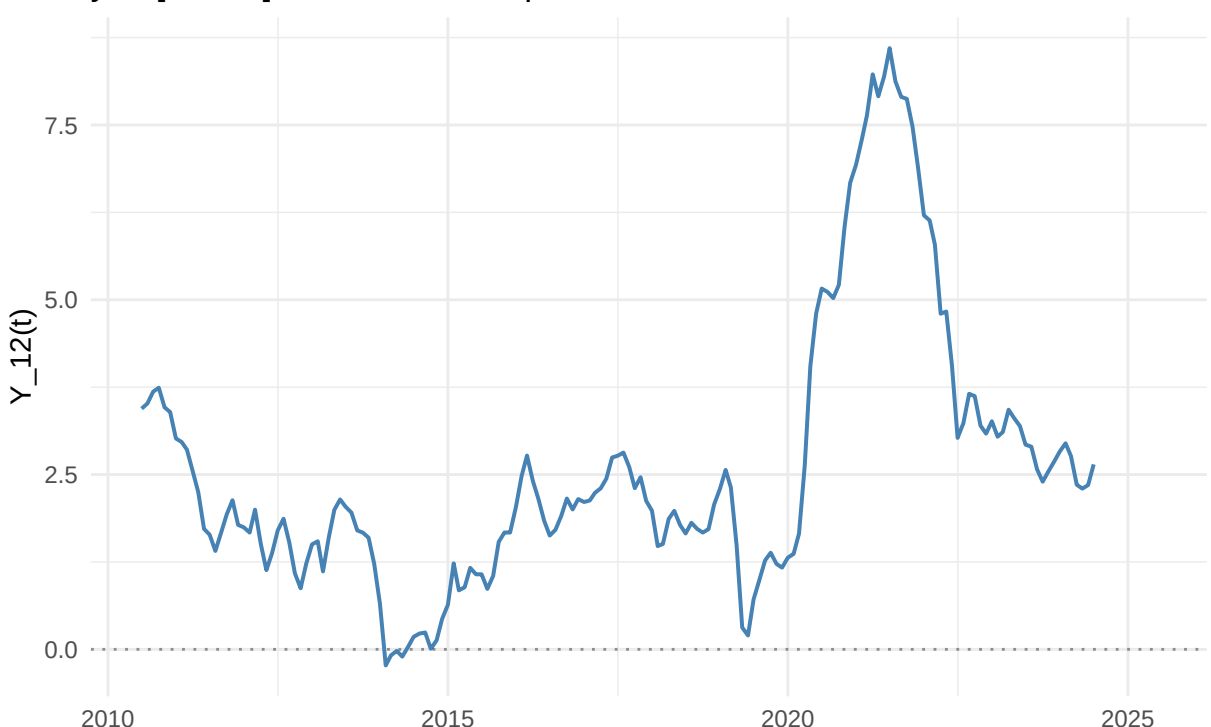
yout[, h=12]: cumulativo 12-passos
