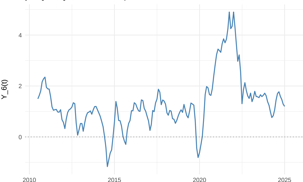
yout[, h=6]: cumulativo 6-passos
