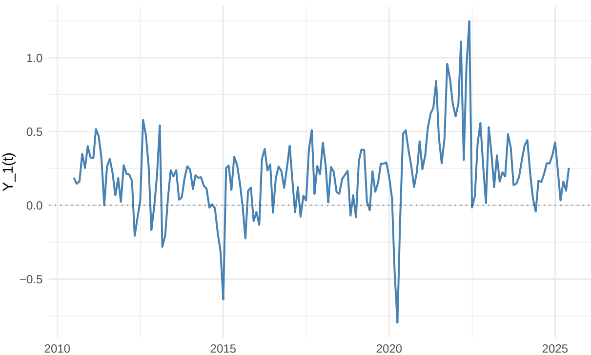
yout[, h=1]: cumulativo 1-passos
