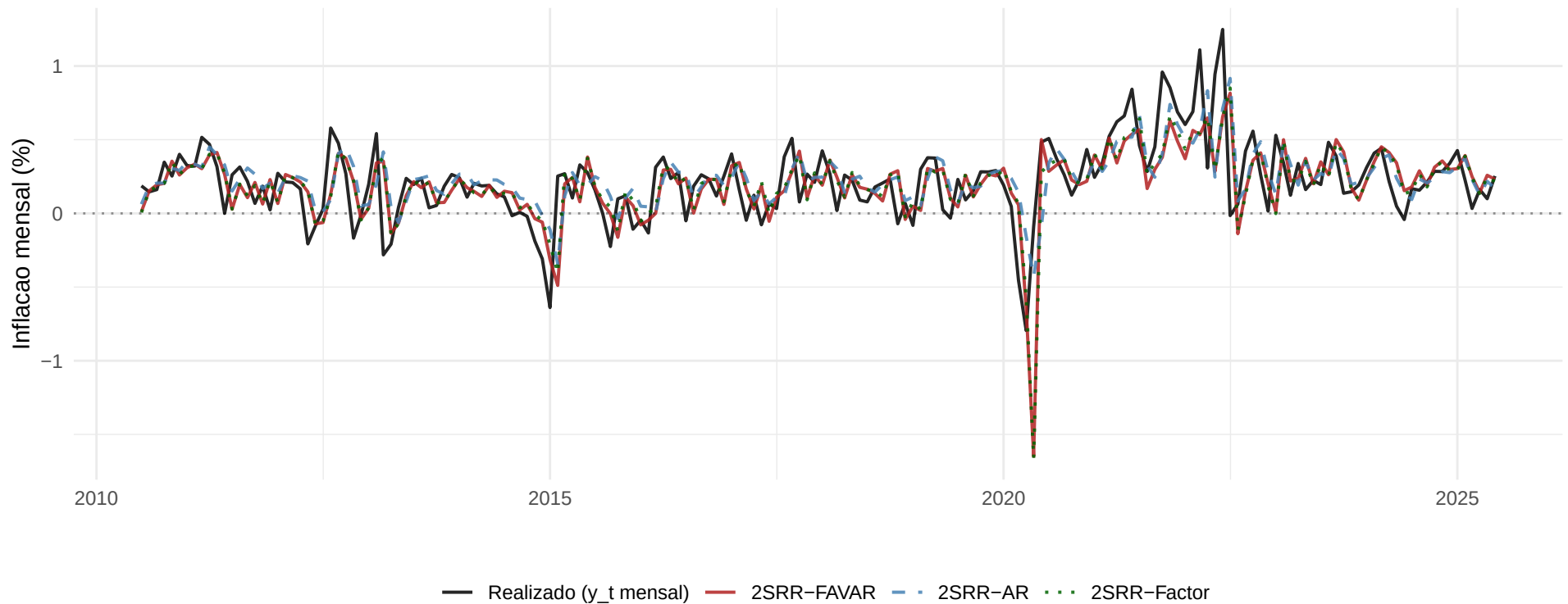
2SRR (3 casos) vs Realizado mensal, h=1
