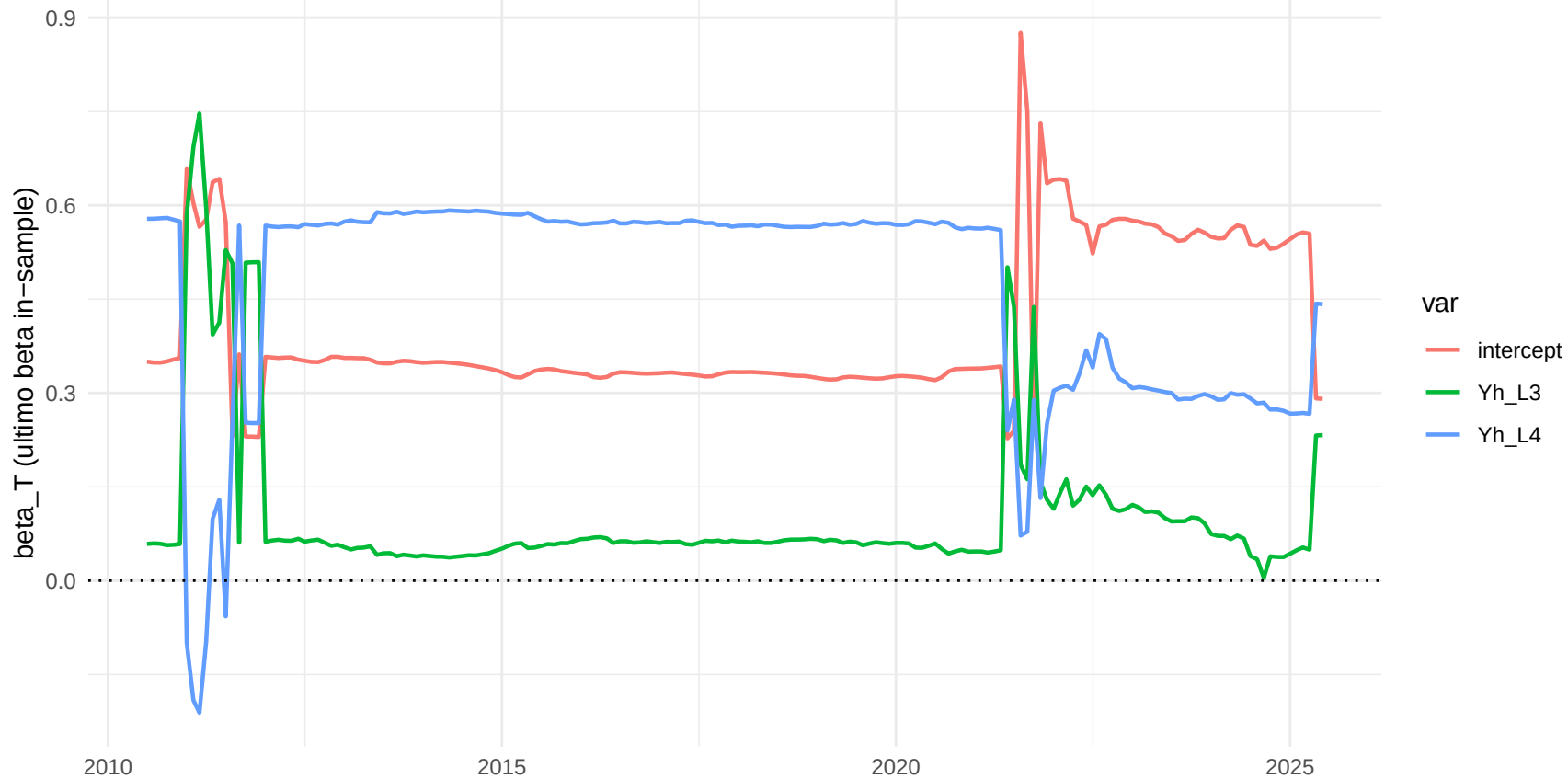
TVP-AR, h=3: top-3 betas (por sd)
