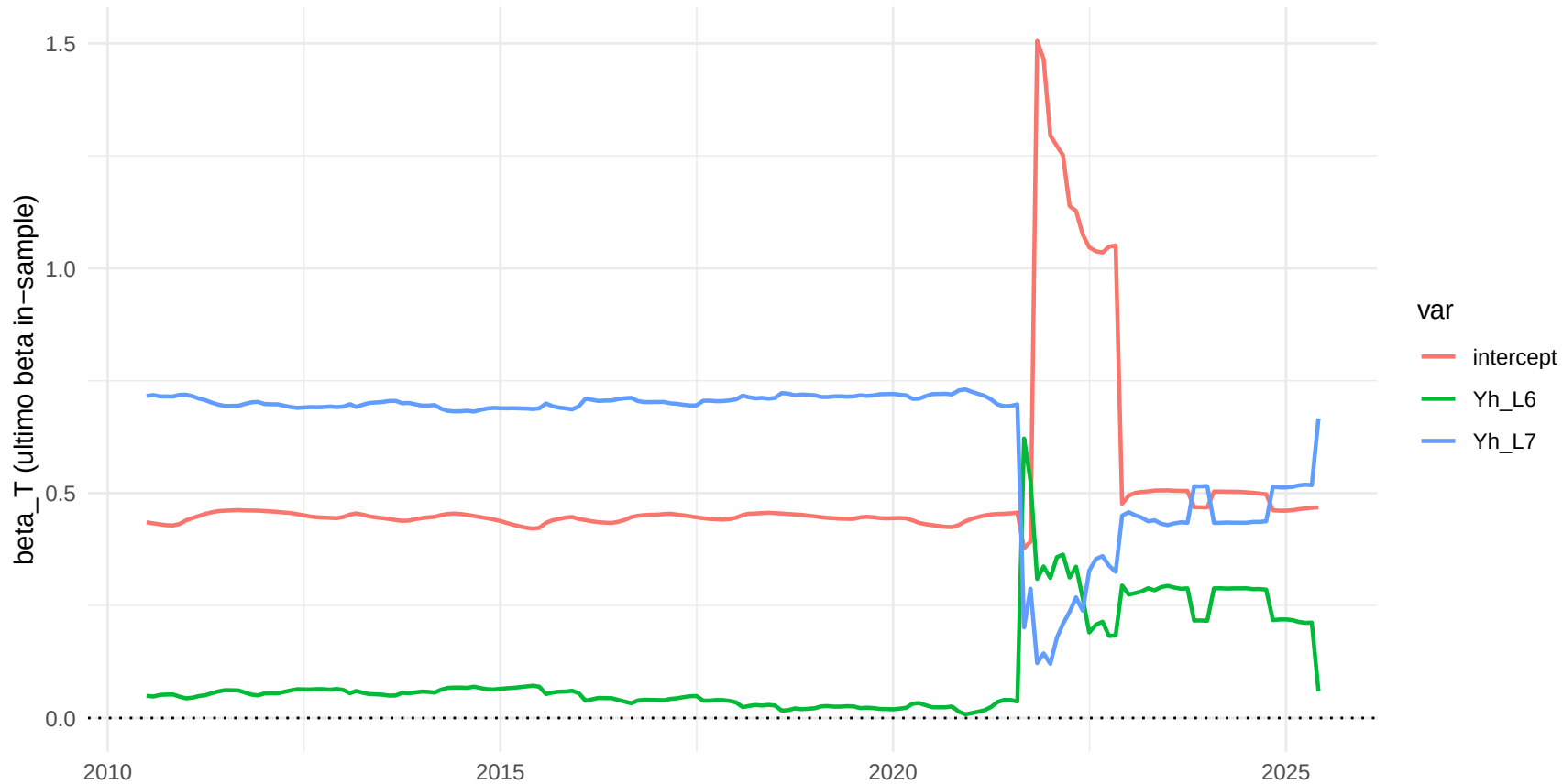
TVP-AR, h=6: top-3 betas (por sd)
