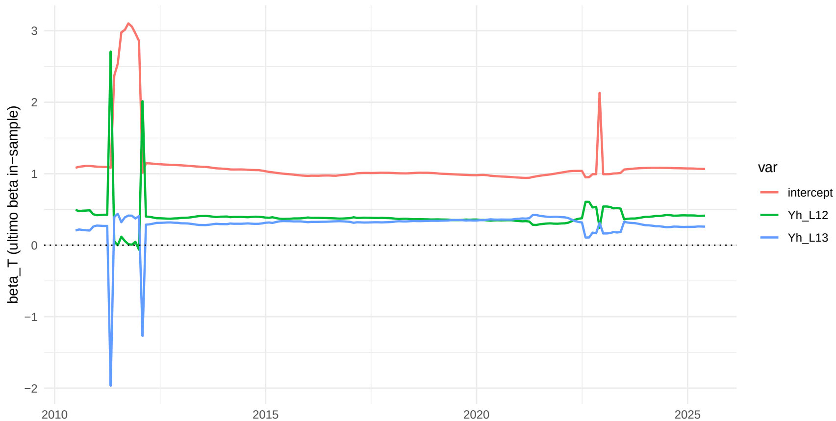
TVP-AR, h=12: top-3 betas (por sd)
