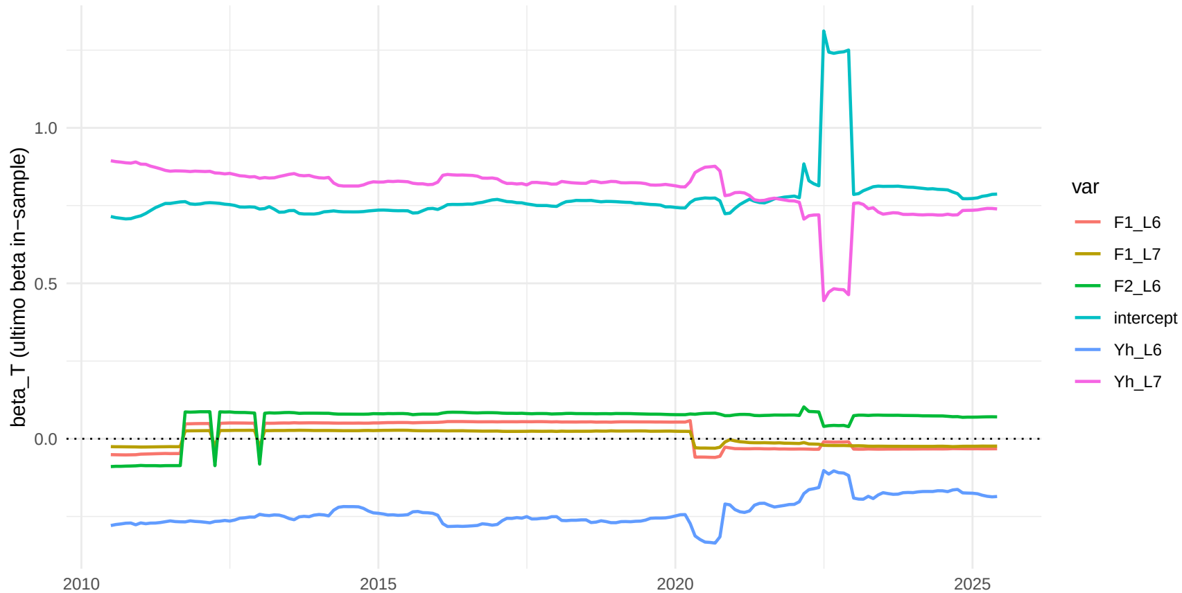
TVP-FAVAR, h=6: top-6 betas (por sd)
