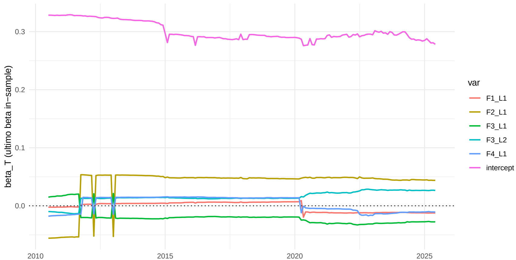
TVP-Factor, h=1: top-6 betas (por sd)
