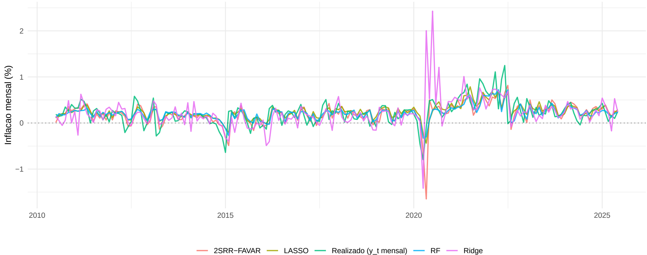
Forecasts h=1 (escala mensal): 2SRR-FAVAR + 2 melhores + pior Medeiros
