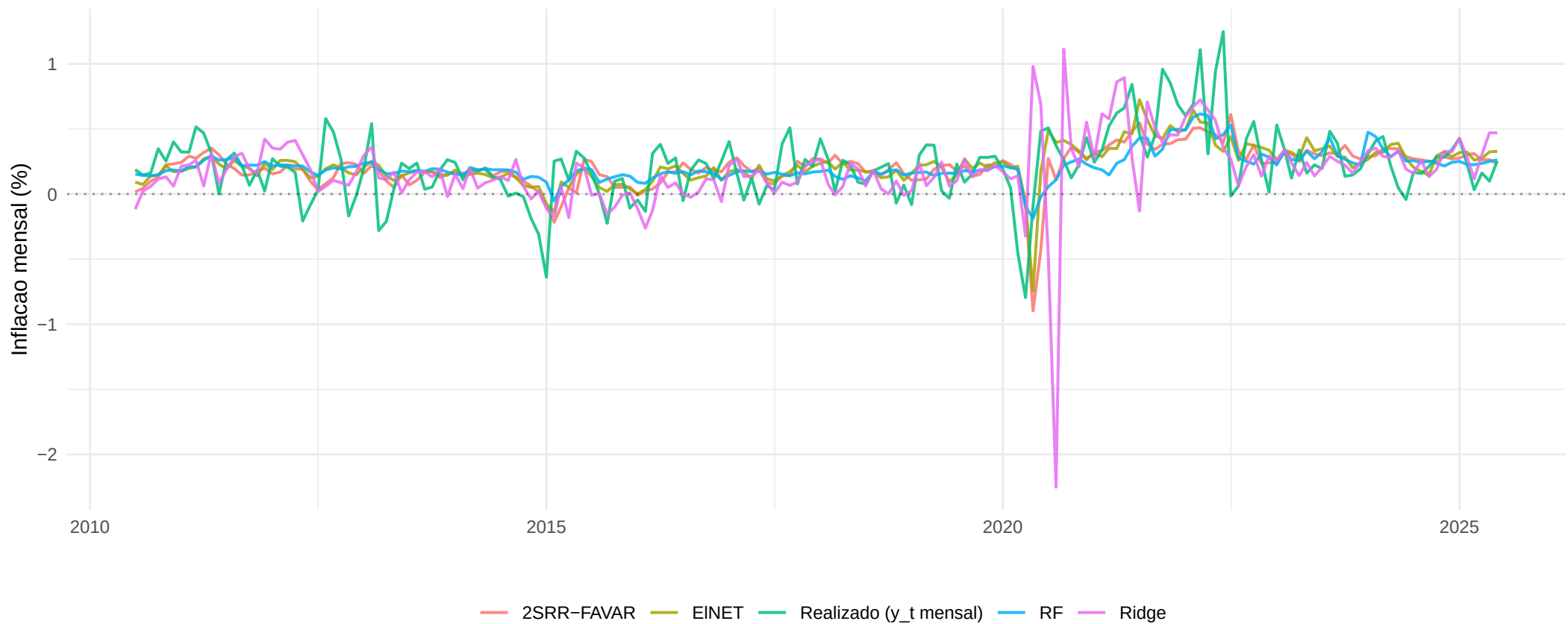
Forecasts h=3 (escala mensal): 2SRR-FAVAR + 2 melhores + pior Medeiros
