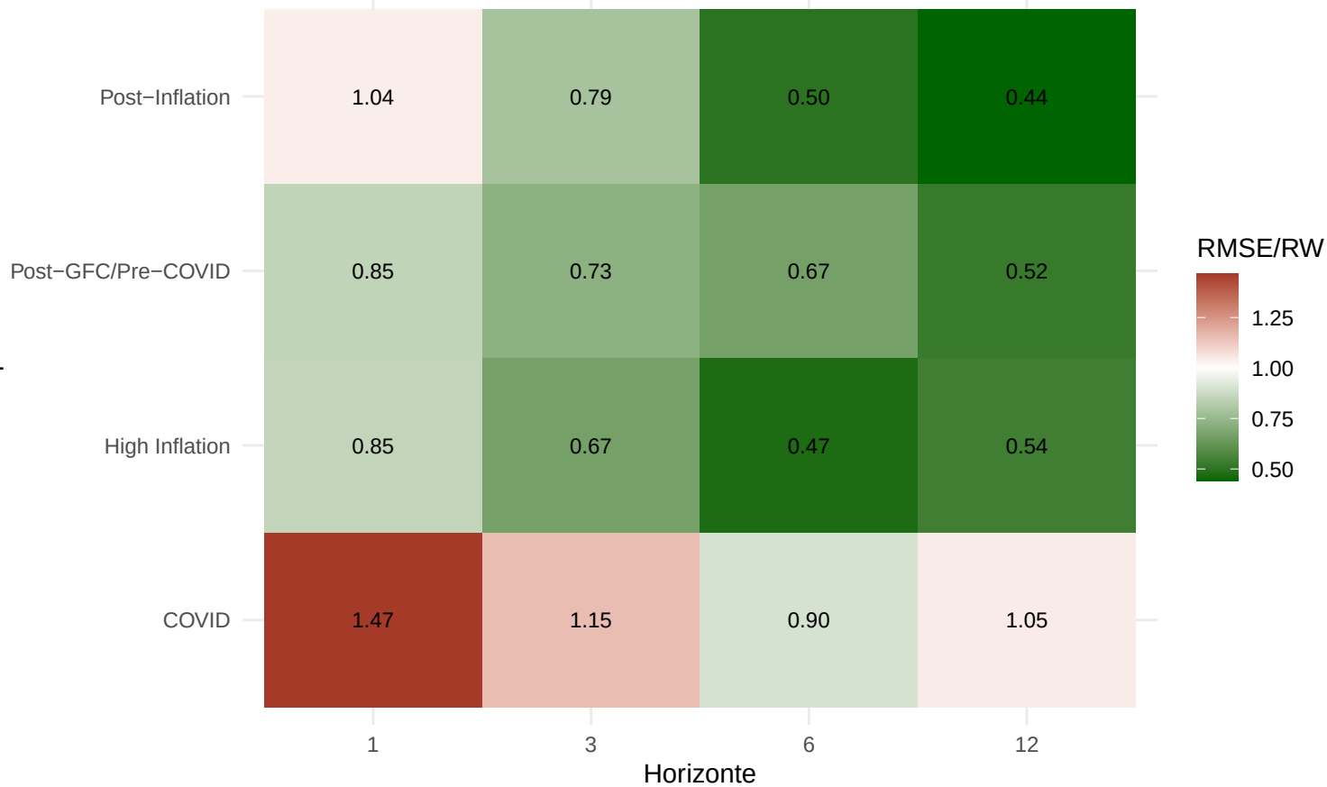
TVP-FAVAR: RMSE relativo ao RW por sub-período
