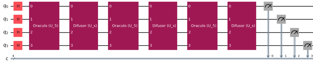
Figura 11: Circuito principal do Algoritmo de Grover abstraído em blocos modulares. O processo evidencia a inicialização em superposição seguida de 3 iterações consecutivas do Oráculo e Difusor.
