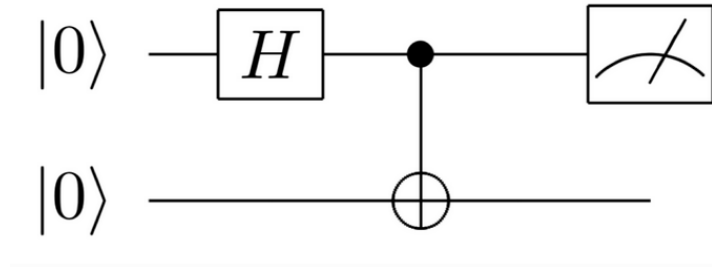
Figura 2: Exemplo de diagrama de circuito quântico. [Qul24]
