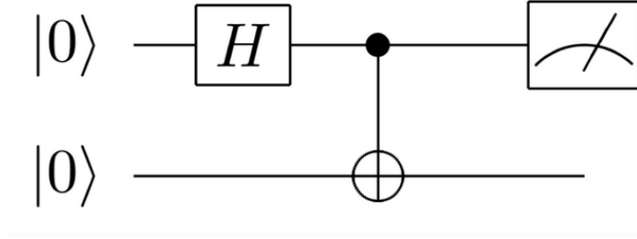
Figura 2: Exemplo de diagrama de circuito quântico. [Qul24]
