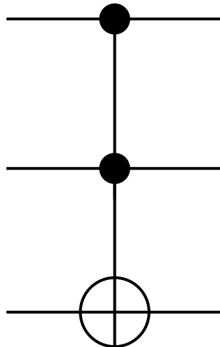
Figura 9: A porta de Toffoli. Se os qbits q_0 e q_1 estiverem no estado |11\rangle uma porta NOT é aplicada em q_2 .
