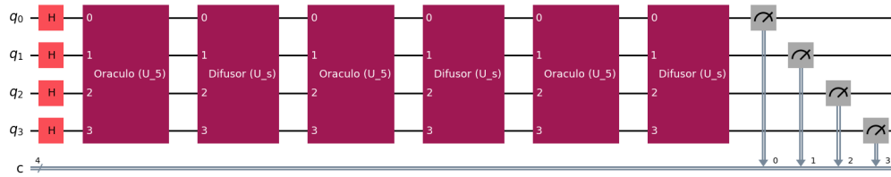
Figura 11: Circuito principal do Algoritmo de Grover abstraído em blocos modulares. O processo evidencia a inicialização em superposição seguida de 3 iterações consecutivas do Oráculo e Difusor.
