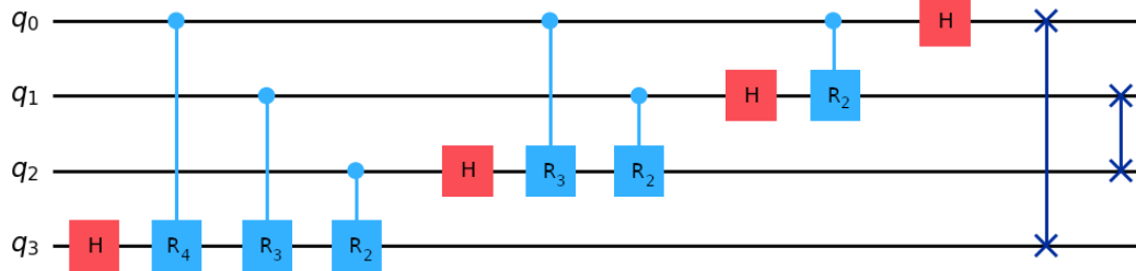
Figura 14: Estrutura do circuito quântico da Transformada de Fourier Quântica (QFT), destacando as portas Hadamard H , as rotações de fase controlada R_k e as portas SWAP finais para reversão da ordem dos qubits.
