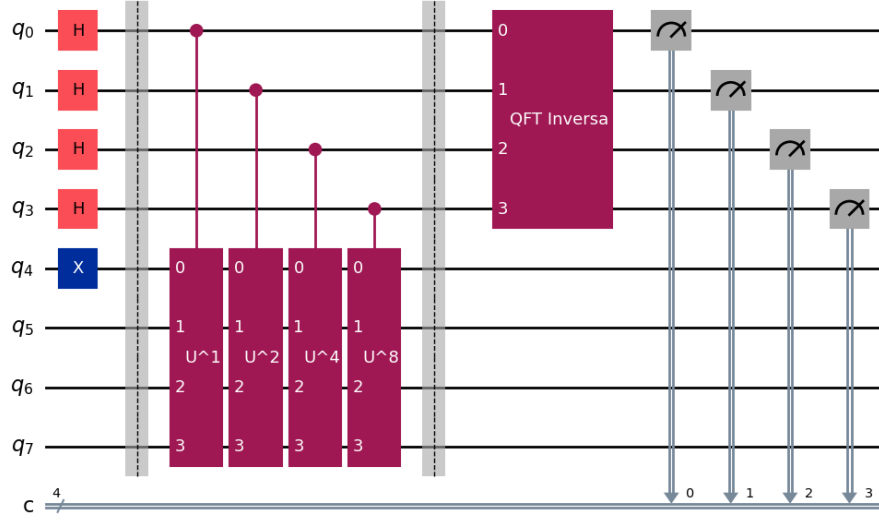
Figura 18: Circuito quântico para busca de período no Algoritmo de Shor ( N = 15 , a = 7 ), integrando a preparação em superposição, as portas modulares controladas U^{2^j} e a Transformada de Fourier Quântica Inversa ( QFT^{-1} ).
