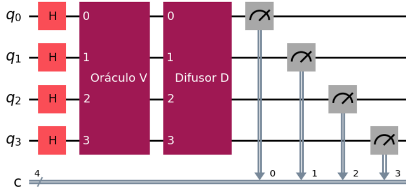
Figura 12: Circuito quântico do Algoritmo BHT estruturado com o operador de superposição H^{\otimes 4} , o oráculo unitário V = F^\dagger U F e o difusor de Householder D , seguido pela medição na base computacional.
