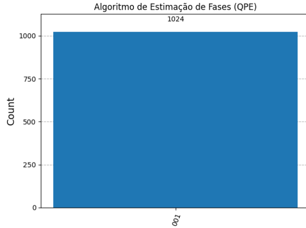
Figura 16: Histograma de resultados da QPE para t = 3 e \theta = 0.125 . A interferência destrutiva suprime a probabilidade de colapso de todos os estados incorretos, isolando a resposta correta.
