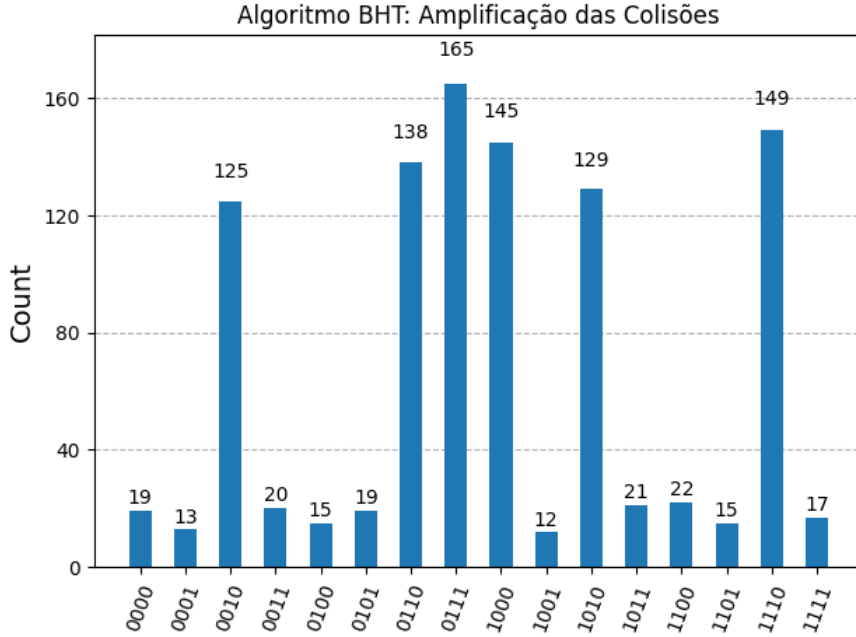
Figura 13: Distribuição de probabilidades obtida no simulador após uma iteração de Grover, evidenciando a amplificação de amplitude dos estados associados às colisões. Como M = 3 no caso N = 16 , devemos ter exatamente 6 estados com a probabilidade amplificada.
