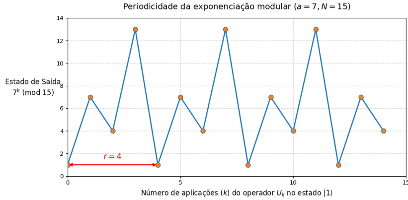
Figura 17: Comportamento periódico da função f(k) = 7^k \pmod{15} . Observa-se que a sequência de estados de saída se repete a cada 4 aplicações do operador, revelando o período r = 4 .
