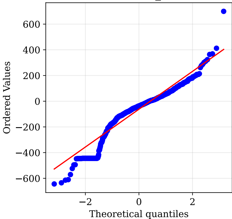
QQ-Plot - svr_model
