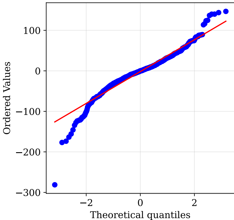
QQ-Plot - BiGRU
