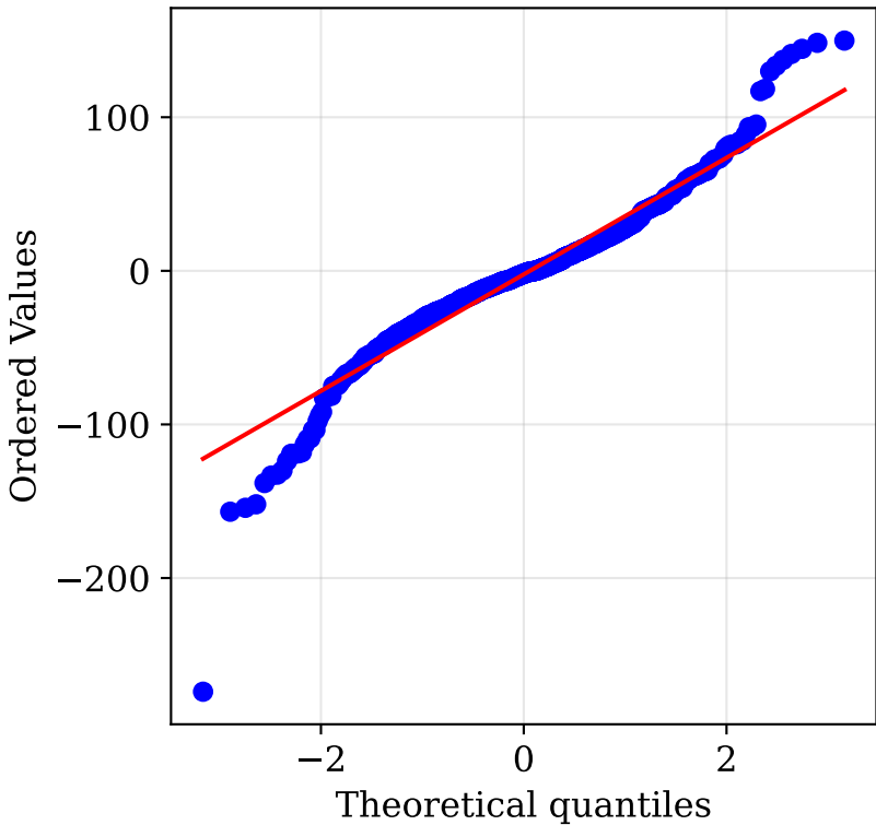
QQ-Plot - gru
