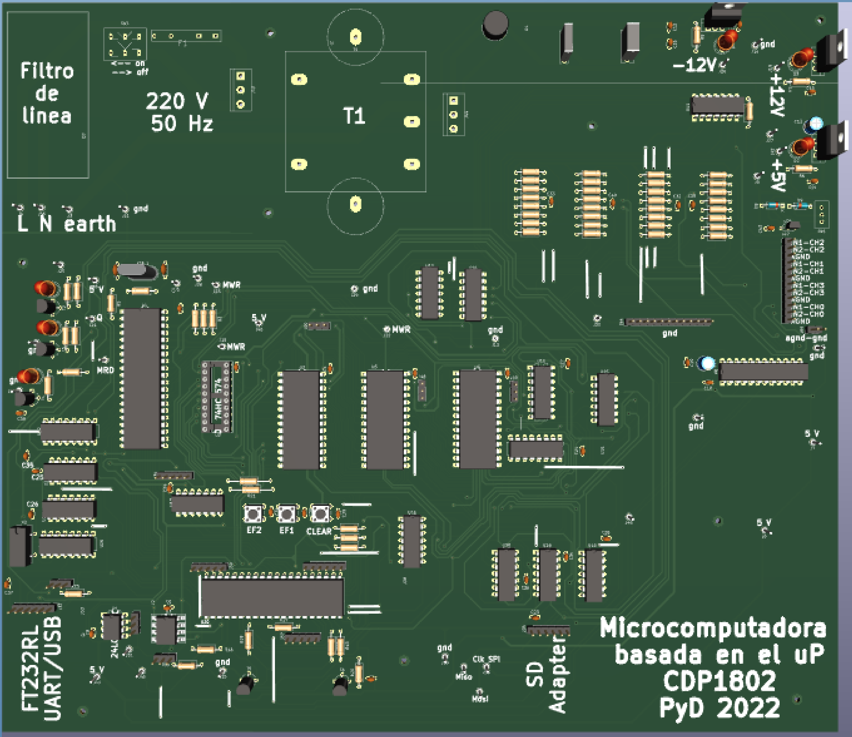
MICROCOMPUTADORA DE USOS GENERALES
