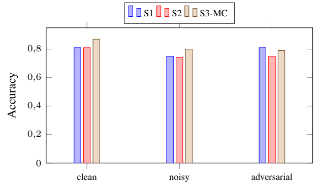
Figura 2: Accuracy bajo corpus limpio, ruidoso y adversarial. S3-MC lidera en clean/noisy, mientras S1 conserva mejor estabilidad relativa en adversarial.
