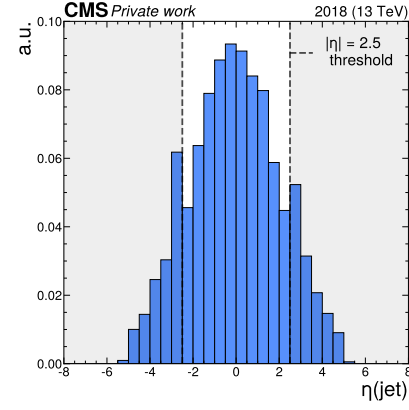
(d) \eta of reconstructed jets.
