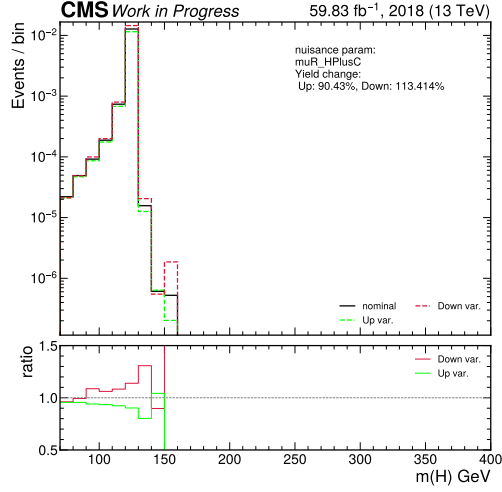
(e) Renormalisation scale: cH(ZZ \rightarrow 4\mu)
