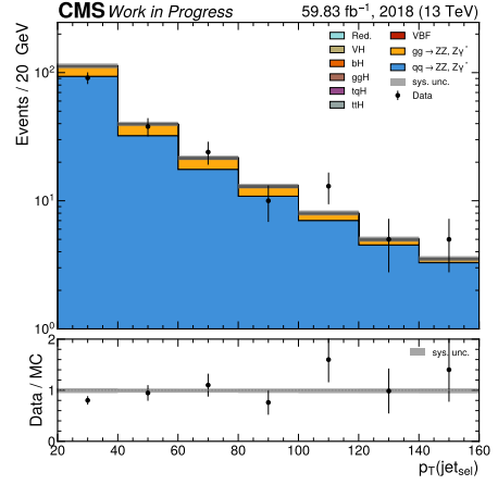
(d) Transverse momentum of the selected jet.
