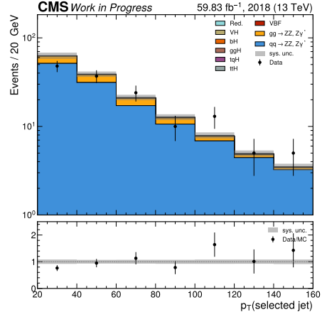
(d) Transverse momentum of the selected jet.
