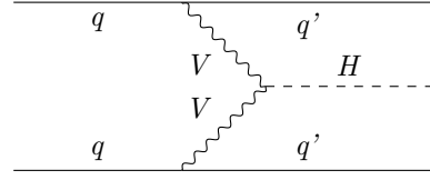
(d) The qqH process.
